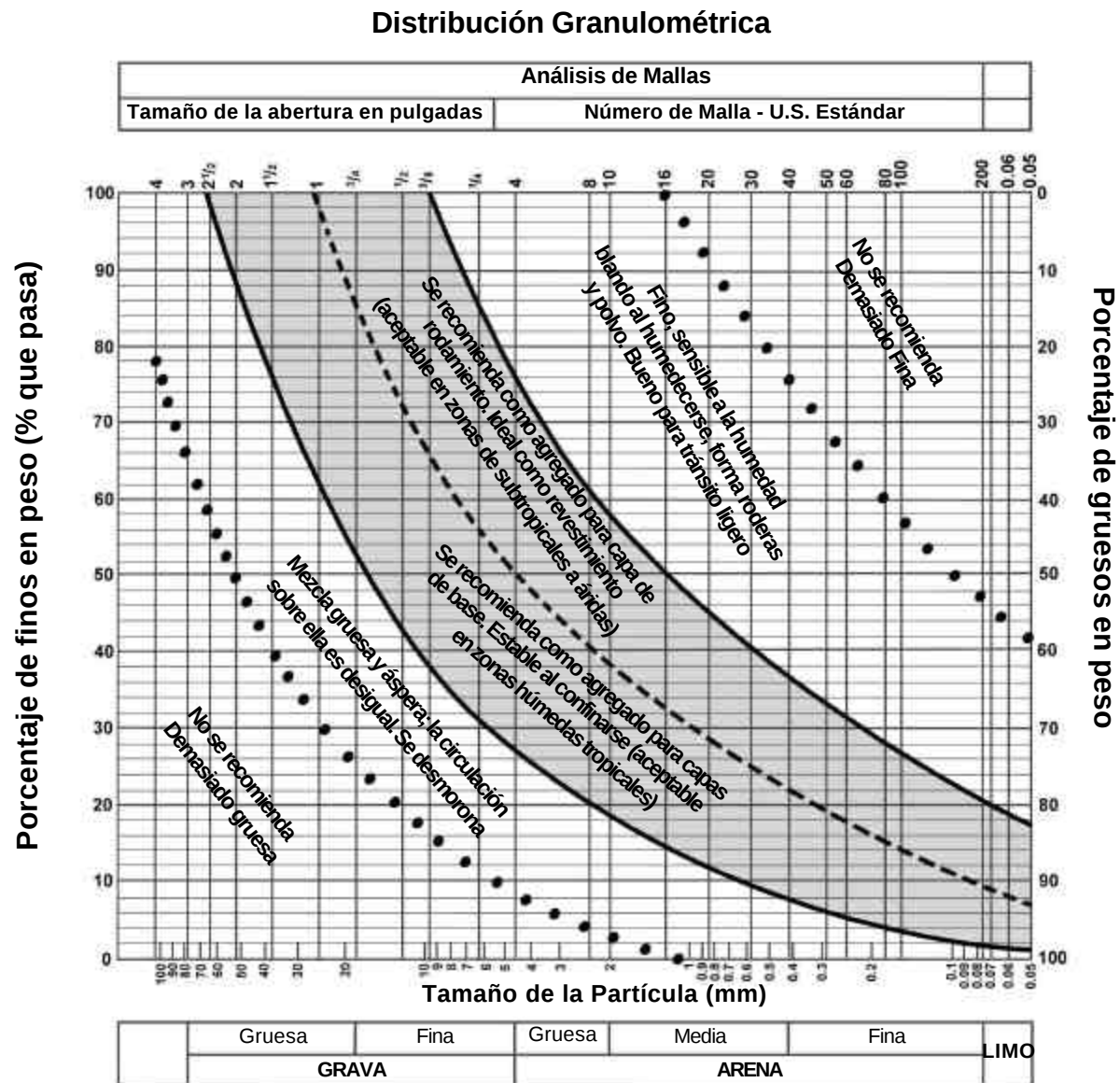
Figura 12.4 Intervalos de variación de la granulometría para amateriales de revestimeinto de caminos y sus características de comportamiento. (Adaptado de R. Charles, 1997 and the Association of Asphalt Paving Technologists)
