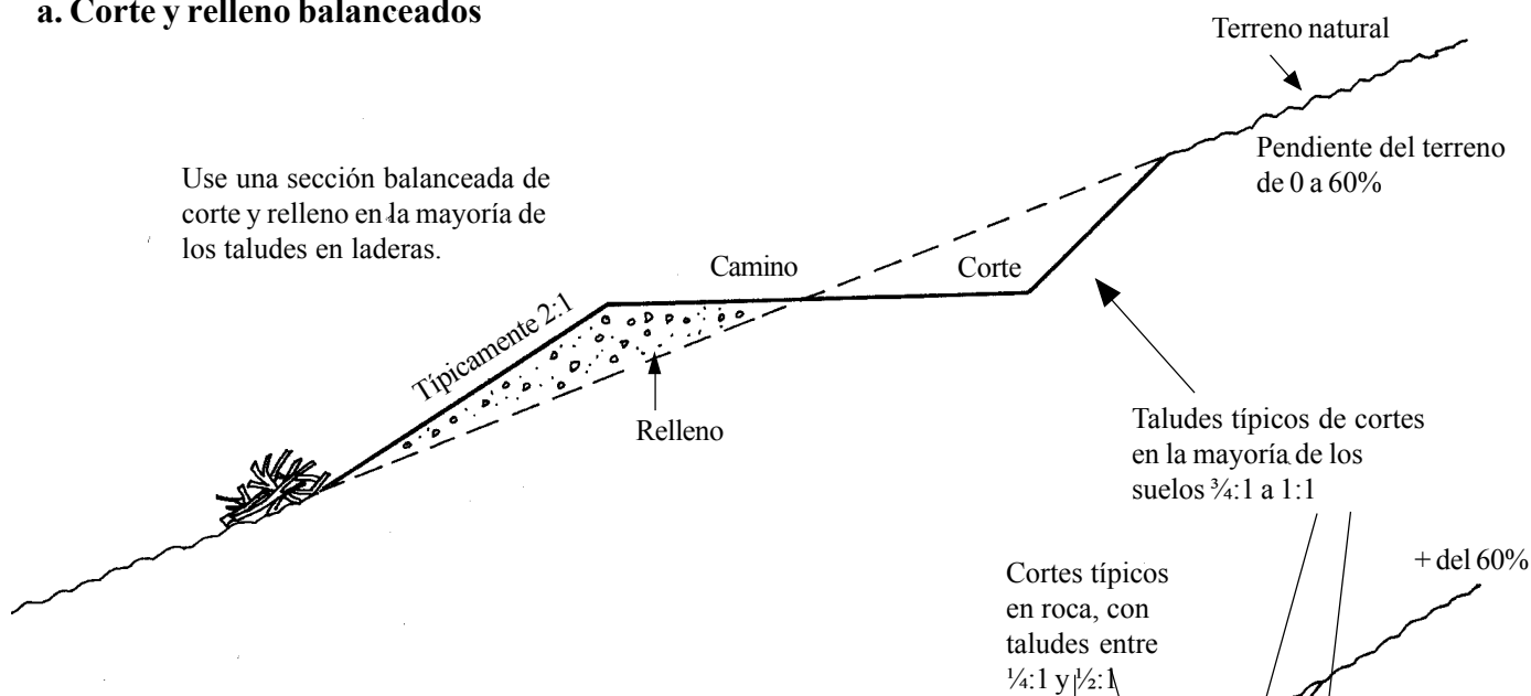
Figura 11.1 Opciones de diseño para taludes de corte.
