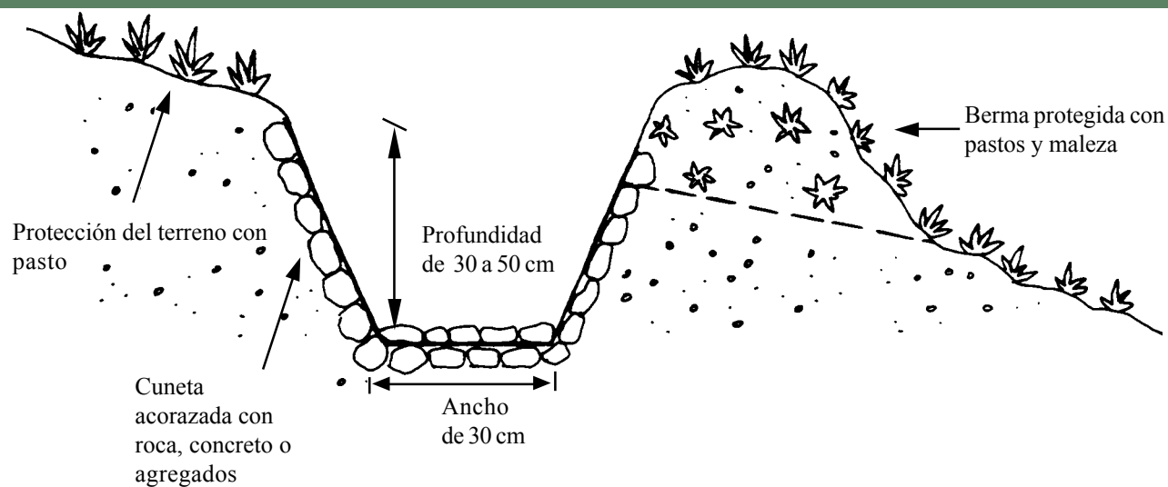
Figura 13.3 Estructuras para el control del agua.
