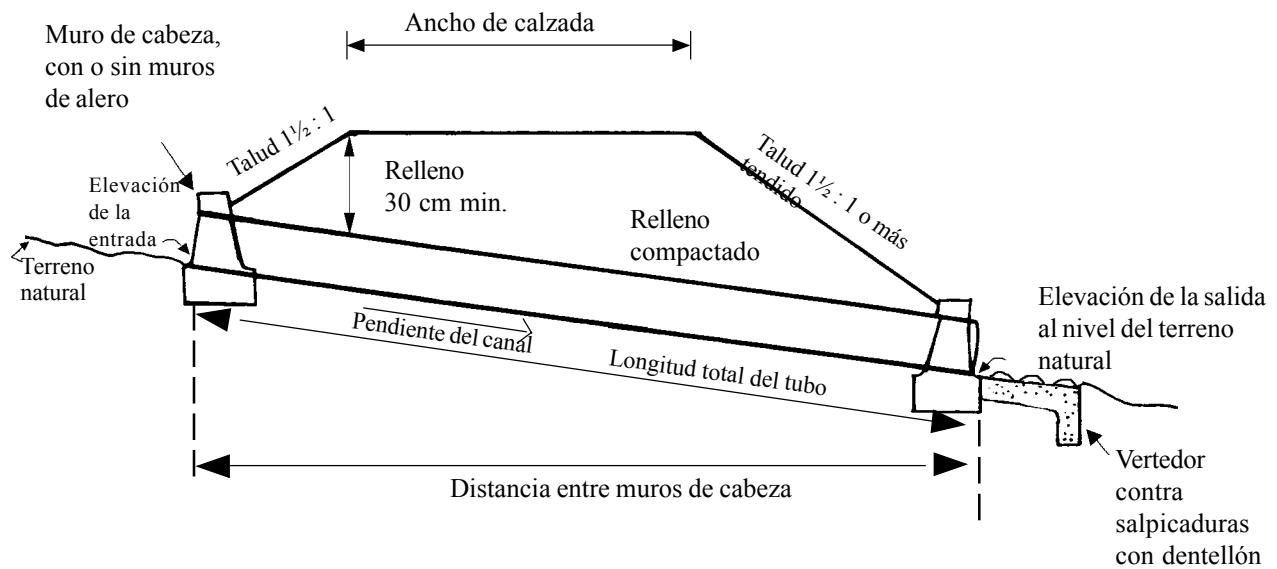
Figura 8.5 Instalación de alcantarillas y detalles de protección de la boca de salida, con vertedores contra salpicaduras o con tanque amortiguador revestido de enrocamiento.
