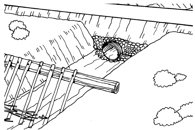
Figura 8.6 Opciones de rejilla en alcantarillas para evitar el taponamiento con escombros. Observe que algunas rejillas están ubicadas en el tubo y otras se localizan aguas arriba del tubo, dependiendo de las condiciones locales y del acceso para limpieza y mantenimiento.
