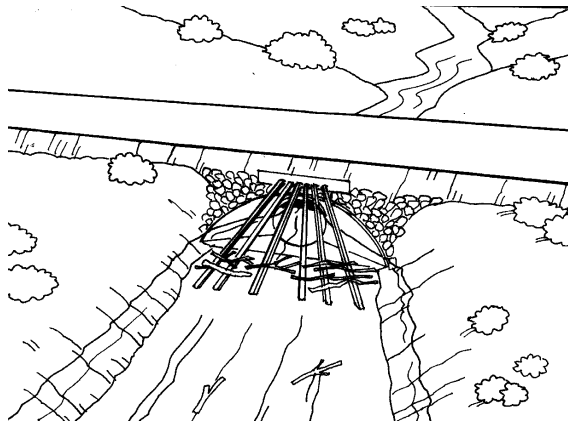
Figura 8.6 Opciones de rejilla en alcantarillas para evitar el taponamiento con escombros. Observe que algunas rejillas están ubicadas en el tubo y otras se localizan aguas arriba del tubo, dependiendo de las condiciones locales y del acceso para limpieza y mantenimiento.
