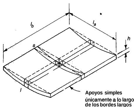
FIGURA 12.2 Forma deflectada de una losa en una dirección y cargada uniformemente.
