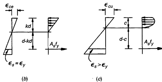
FIGURA 11.11 Características de una rótula plástica en un elemento de concreto reforzado: (a) diagrama típico momento-rotación; (b) deformaciones unitarias y esfuerzos al inicio de la fluencia; (c) deformaciones unitarias y esfuerzos en la falla incipiente.
