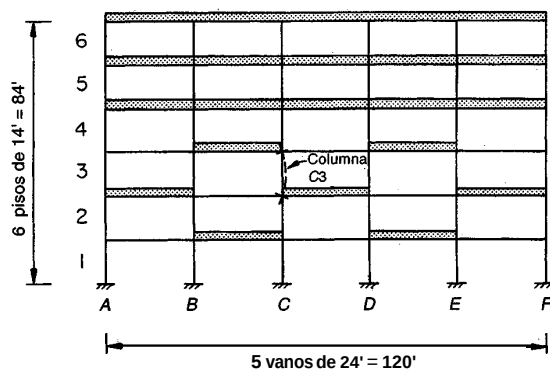
FIGURA 9.14 Pórtico de concreto del edificio del ejemplo 9.1.
