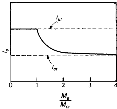
FIGURA 6.4 Variación de I_e , con la relación de momentos.
