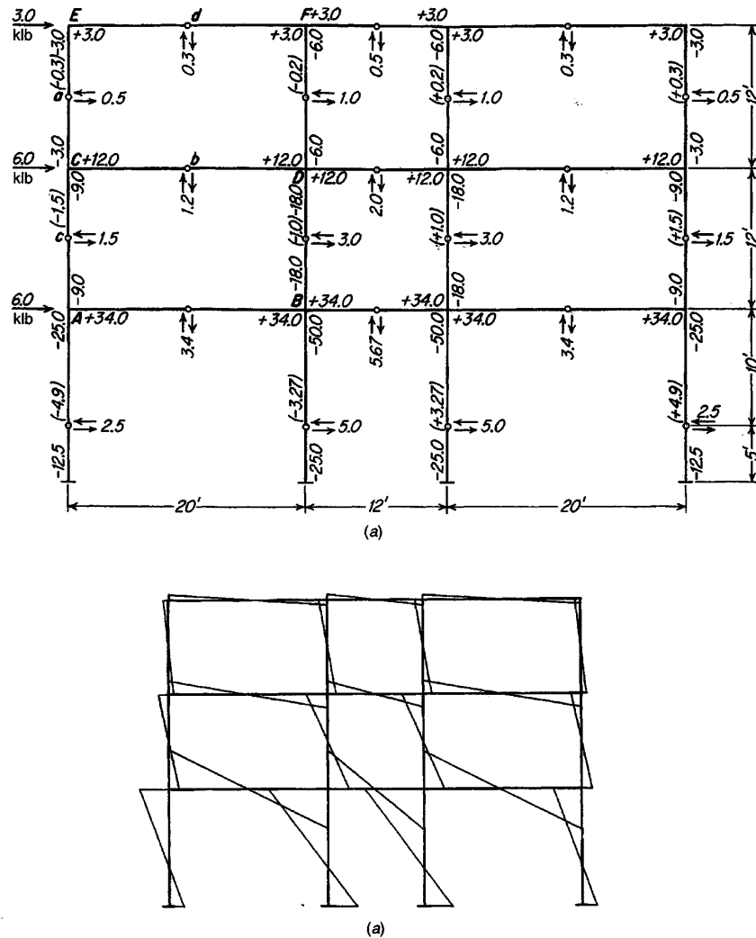
FIGURA 11.7 Método del portal para determinar momentos generados por cargas de viento en un pórtico de edificio: (a) momentos, cortantes y fuerzas axiales; (b) variaciones de los momentos.
