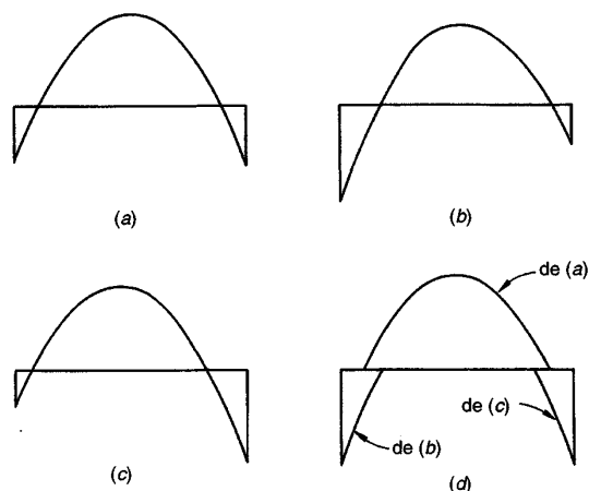
FIGURA 11.9 Diagramas de momentos máximos y envolvente de momentos para vigas continuas: (a) momento positivo máximo; (b) momento negativo máximo en el extremo izquierdo; (c) momento negativo máximo en el extremo derecho; (d) envolvente de momentos.
