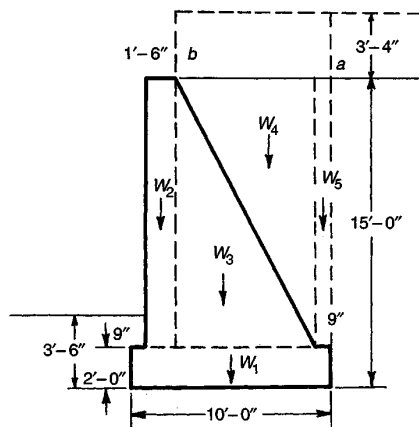
FIGURA 17.6 Muro de contención de gravedad.
