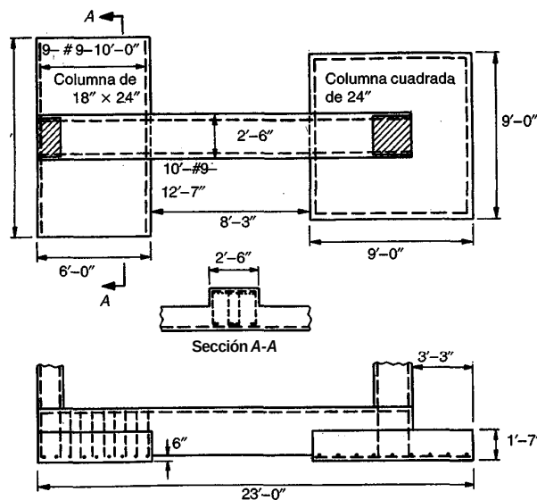
FIGURA 16.18 Zapatas con viga de amarre del ejemplo 16.4.
