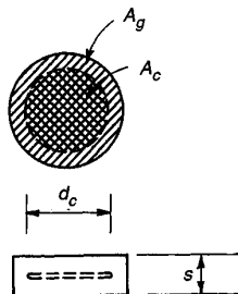
FIGURA 8.6 Confinamiento del núcleo de concreto a causa de la tensión circular.
