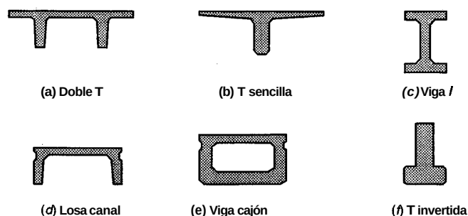
FIGURA 19.18 Secciones transversales típicas para vigas.
