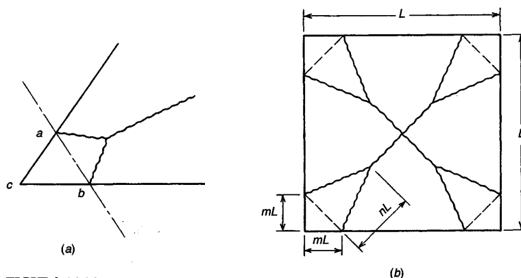
FIGURA 14.14 Condiciones de las esquinas.
