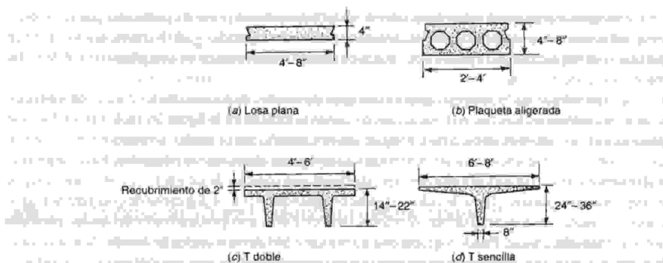
FIGURA 18.16 Elementos prefabricados de cubierta y de entrepiso.
