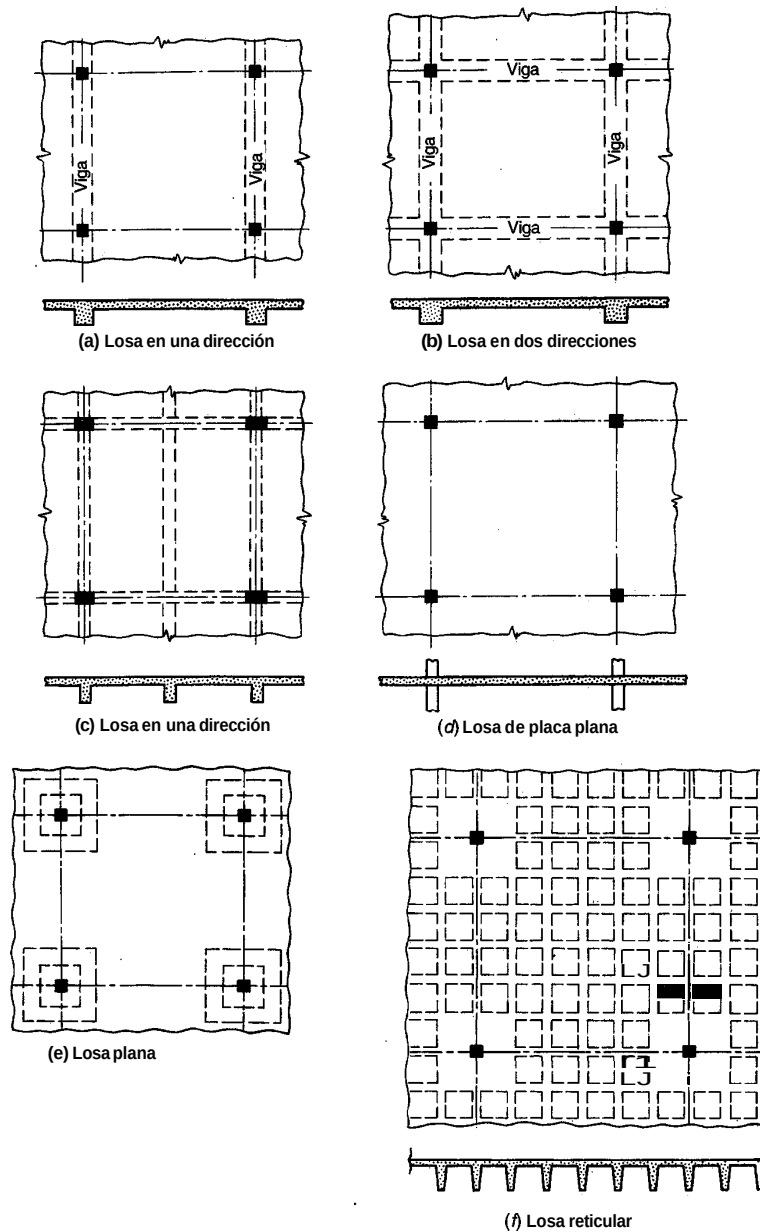
FIGURA 12.1 Tipos de losas estructurales.
