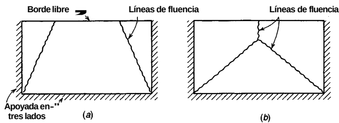
FIGURA 14.5 Mecanismos alternos para una losa apoyada en tres lados.
