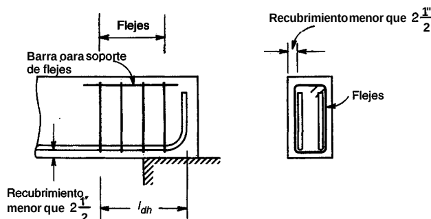
FIGURA 5.11 Requisitos de refuerzo transversal en extremos discontinuos de elementos con recubrimientos pequeños.
