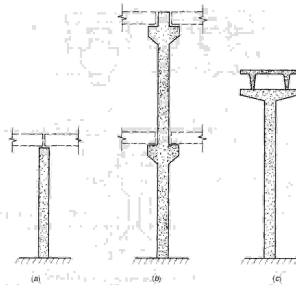
FIGURA 18.18 Columnas prefabricadas de concreto.
