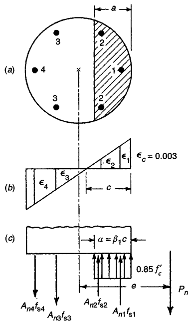
FIGURA 8.13 Columna circular sometida a compresión más flexión.
