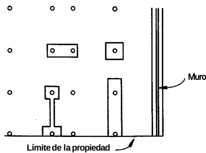
FIGURA 16.1 Tipos de zapatas superficiales.
