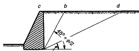
FIGURA 17.2 Bases para la determinación de las presiones de tierra activa y pasiva
