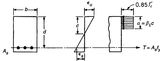
FIGURA 3.9 Viga rectangular simplemente reforzada.
