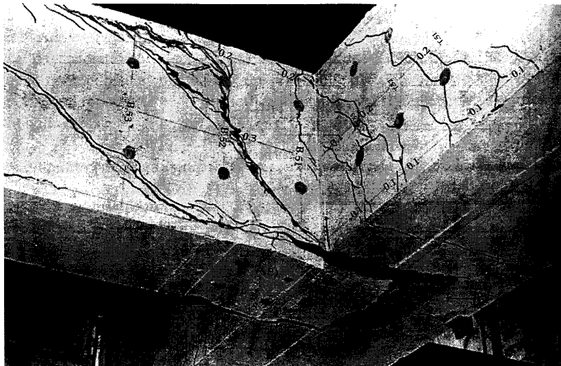
FIGURA 10.14 Falla ocasionada por la falta de soporte para la compresión diagonal en una unión viga secundaria-viga principal.
