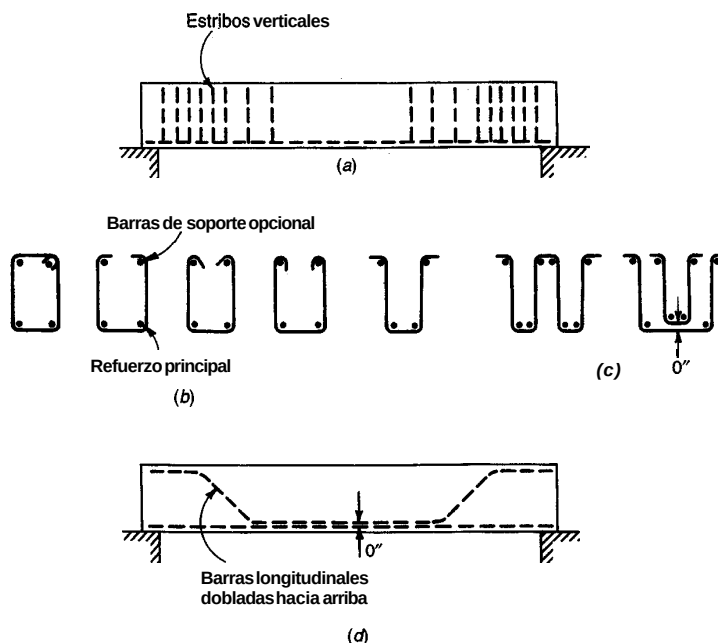
FIGURA 4.8 Tipos de refuerzo en el alma.
