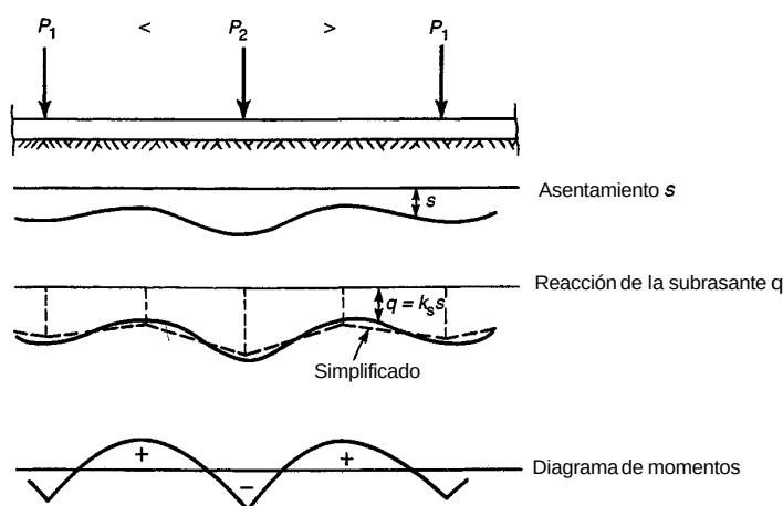
FIGURA 16.20 Zapata continua ( adaptada de la referencia 16.7 ).
