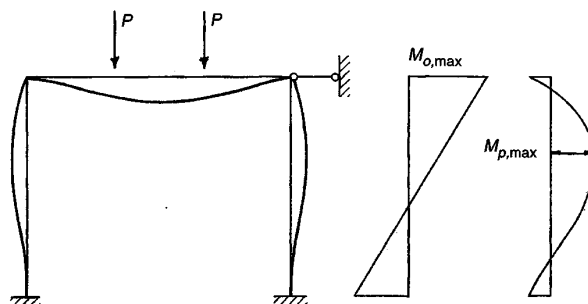
FIGURA 9.9 Pórtico empotrado y arriostrado lateralmente.
