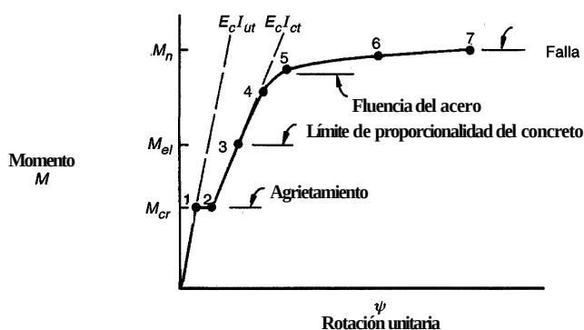
FIGURA 6.16 Relación momento-curvatura para vigas reforzadas a tensión.
