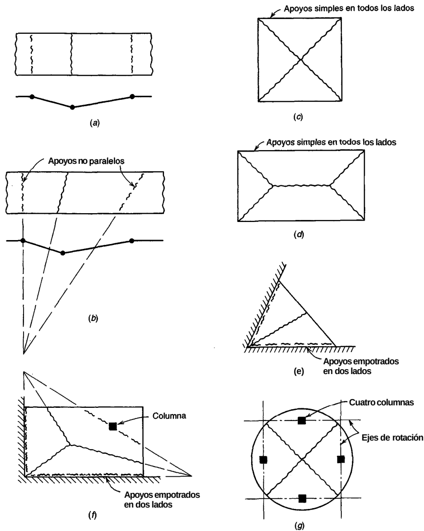
FIGURA 14.4 Patrones comunes de línea de fluencia.
