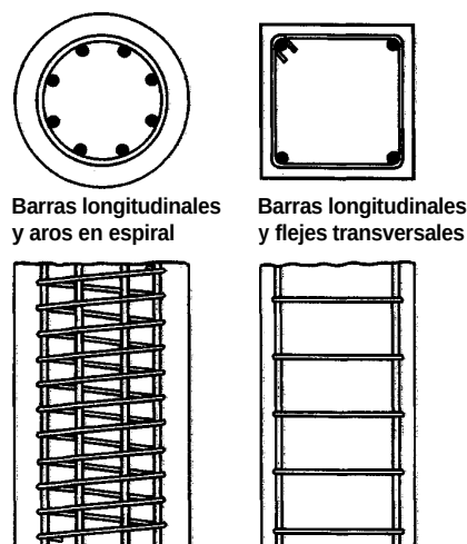
FIGURA 1.14 Columnas de concreto reforzado.
