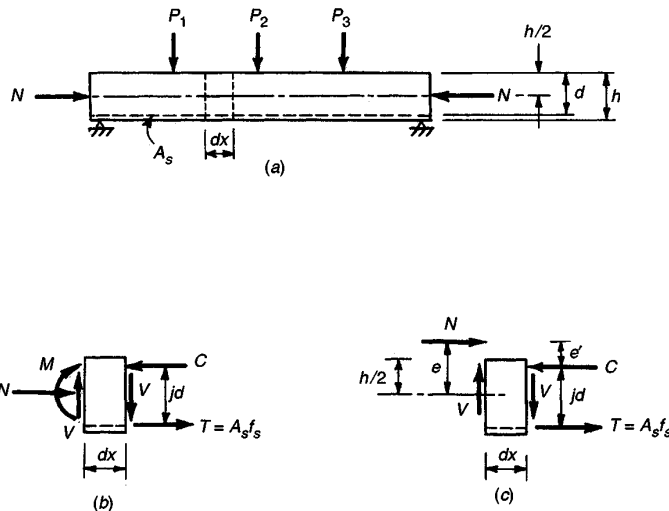
FIGURA 4.15 Vigas sometidas a compresión axial, más cargas de flexión y cortante.
