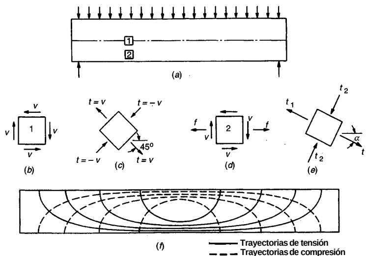
FIGURA 4.3 Trayectorias de esfuerzos en vigas rectangulares homogéneas.
