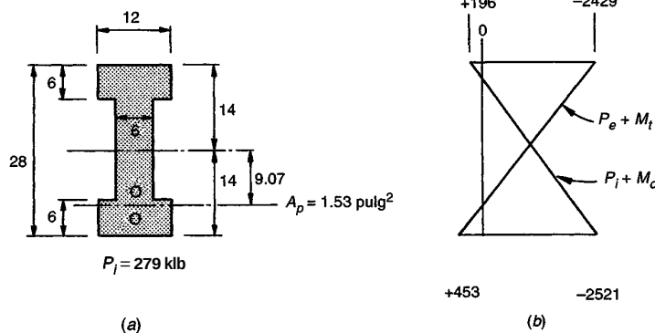
FIGURA 19.15 Ejemplo de diseño de una viga con tendones de excentricidad variable: (a) dimensiones de la sección transversal; (b) esfuerzos en el concreto en el centro de la luz.
