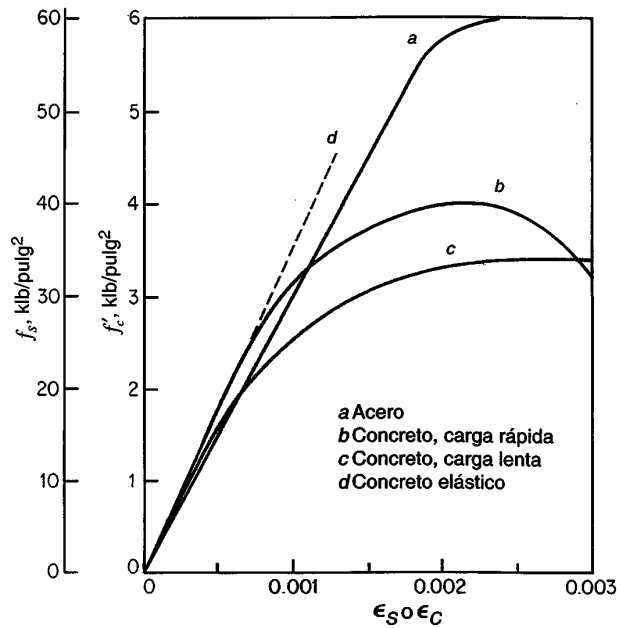
FIGURA 1.15 Curvas de esfuerzo en concreto y acero.
