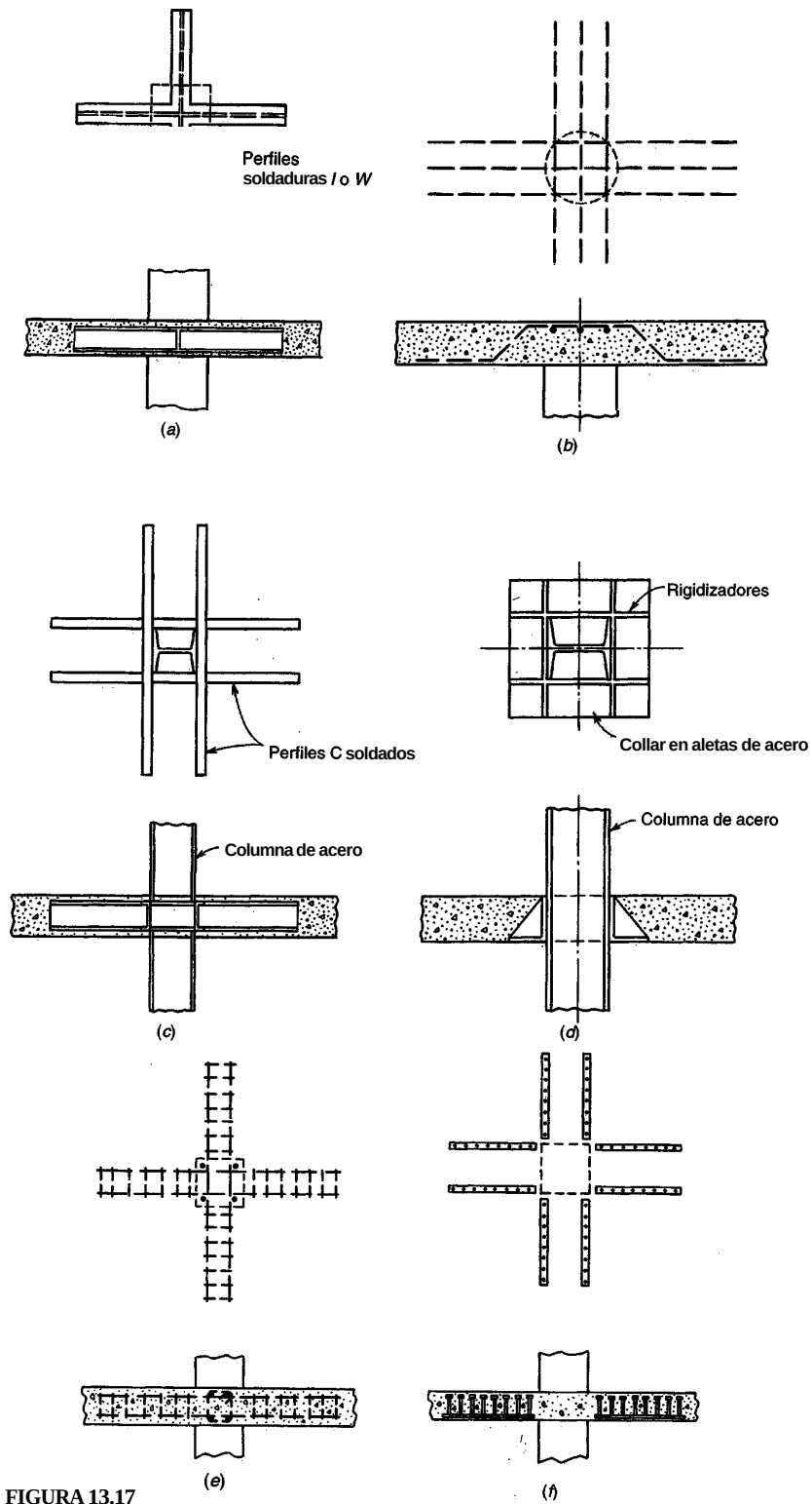
FIGURA 13.17 Refuerzo a cortante para placas planas.
