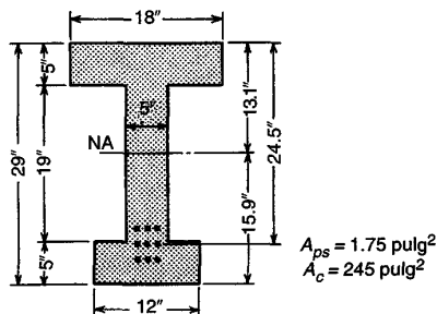
FIGURA 19.24 Viga postensada del ejemplo 19.6.
