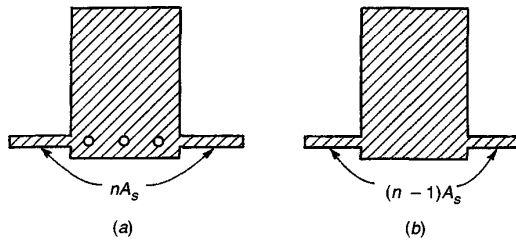
FIGURA 3.3 Sección transformada no fisurada de una viga.
