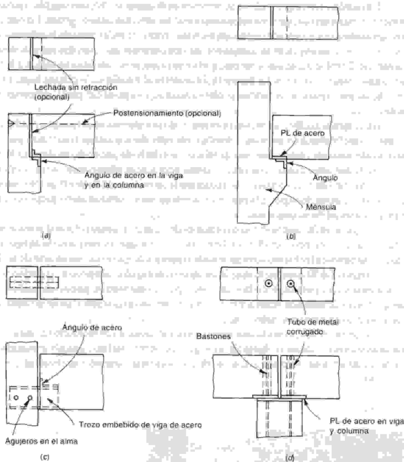
FIGURA 18.30 Conexiones de vigas a columnas.
