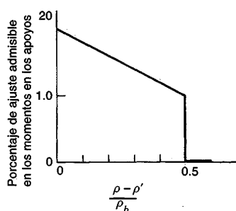
FIGURA 11.15 Redistribución de momentos permitida por el Código ACI.
