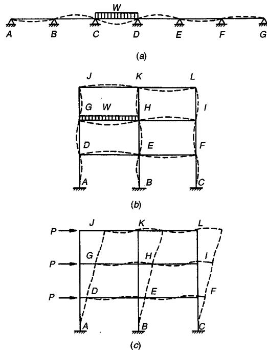
FIGURA 11.1 Forma deflectada de vigas y pórticos continuos.
