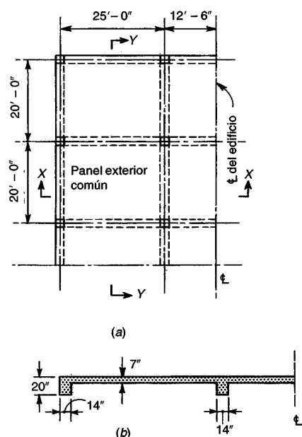
FIGURA 13.9 Losa de piso en dos direcciones con vigas en los ejes de columnas: (a) planta parcial del piso; (b) sección X-X (la sección Y-Y es similar).
