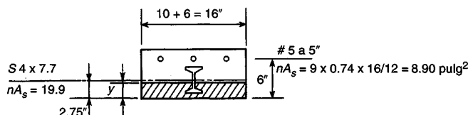
FIGURA 13.21 Sección efectiva de la losa.
