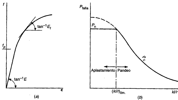
FIGURA 9.2 Efecto de la esbeltez sobre la resistencia de columnas cargadas axialmente.
