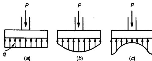
FIGURA 16.2 e presiones de contacto: (a) supuesta; (b) real para suelos granulares; (c) real para suelos cohesivos.
