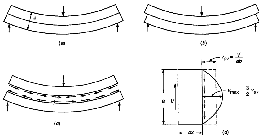
FIGURA 4.2 Cortante en vigas rectangulares homogéneas.
