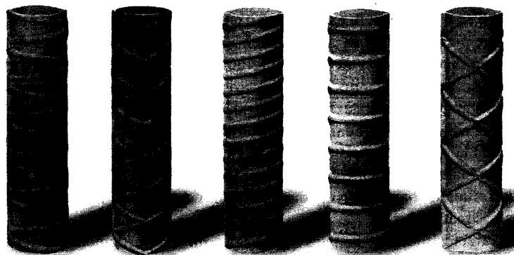
FIGURA 2.12 Tipos de barras de refuerzo corrugadas.
