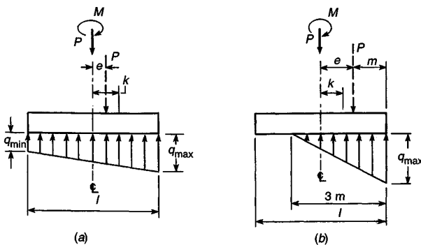
FIGURA 16.3 Presiones de contacto supuestas bajo zapatas excéntricas.
