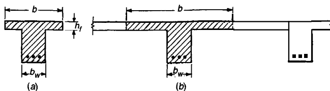
FIGURA 3.13 Ancho efectivo del ala en vigas T.
