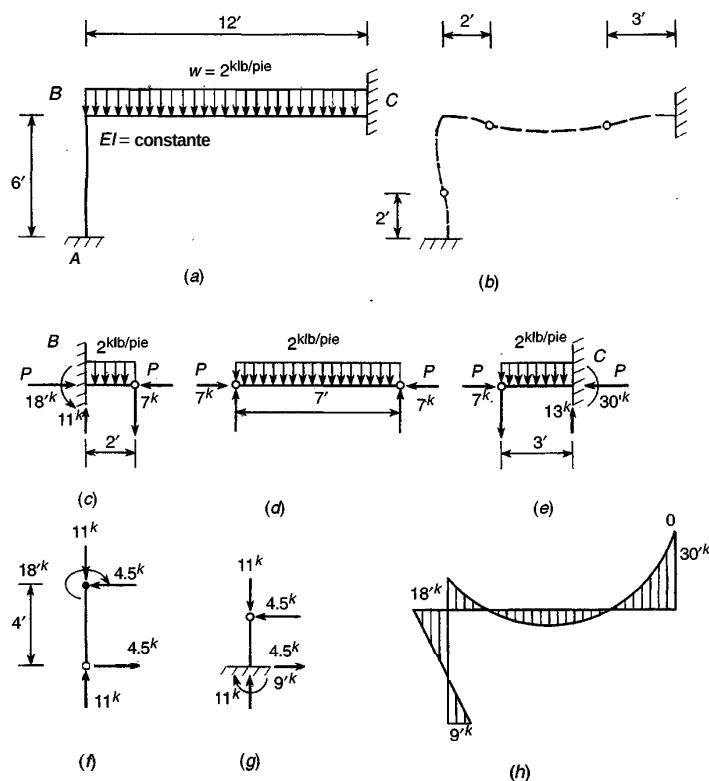
FIGURA 11.6 Análisis aproximado de un pórtico rígido.
