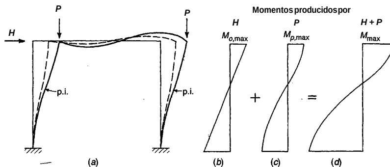
FIGURA 9.8 Pórtico empotrado y sin arriostramiento lateral.
