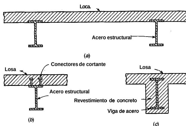
FIGURA 18.5 Entresijos compuestos de viga y losa.
