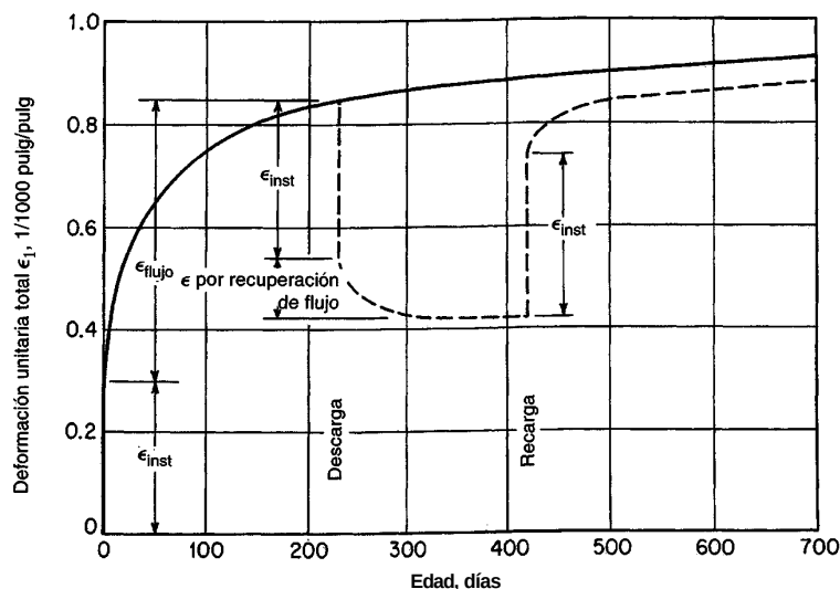
FIGURA 2.7 Curva típica de flujo plástico (concreto sometido a un esfuerzo de 600 \text{ lb/pulg}^2 a una edad de 28 días).
