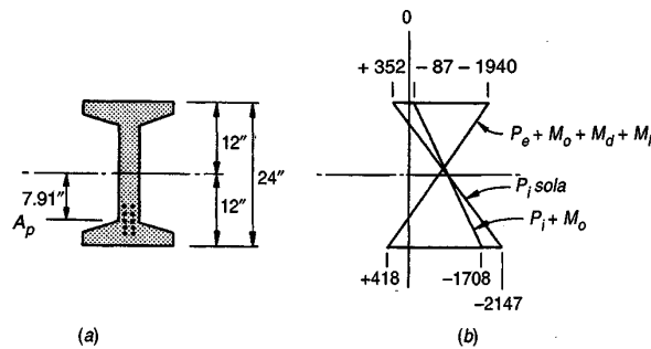
FIGURA 19.12 Ejemplo de diseño: viga I pretensada.
