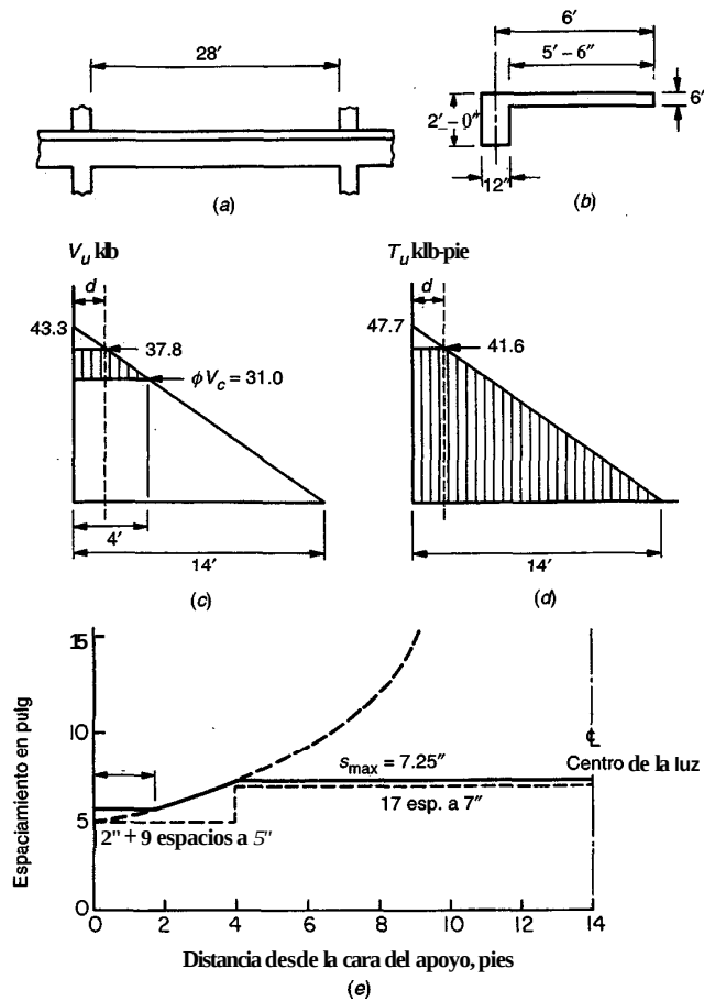
FIGURA 7.12 Ejemplo de diseño para cortante y torsión
