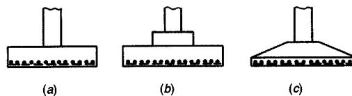
FIGURA 16.5 Tipos de zapatas para columnas individuales.
