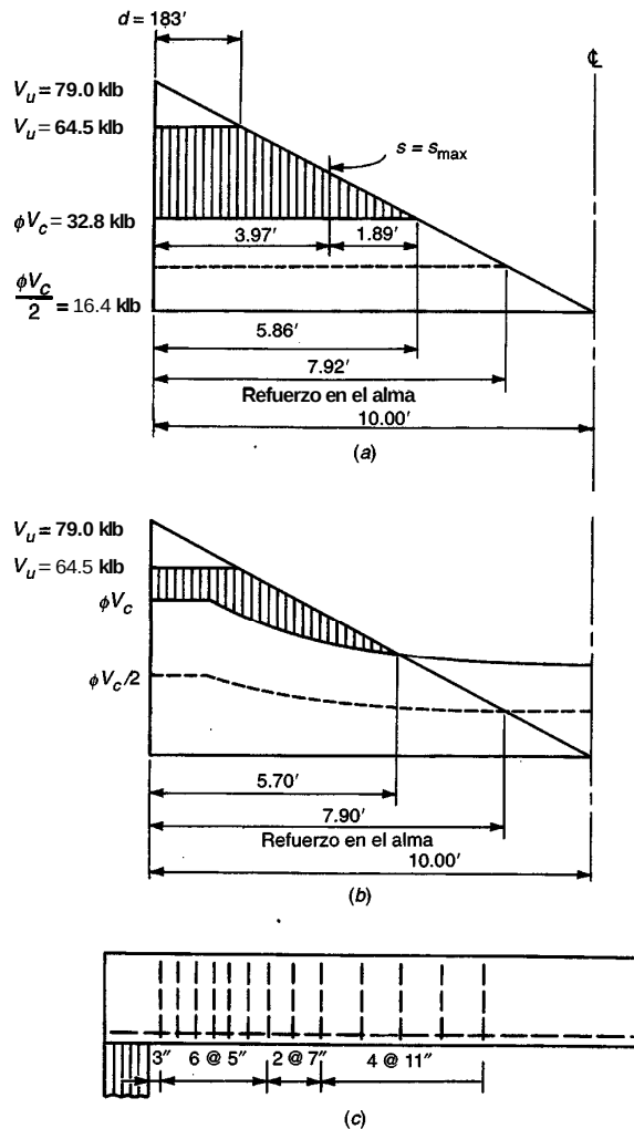
FIGURA 4.12 Ejemplo de diseño a cortante.
