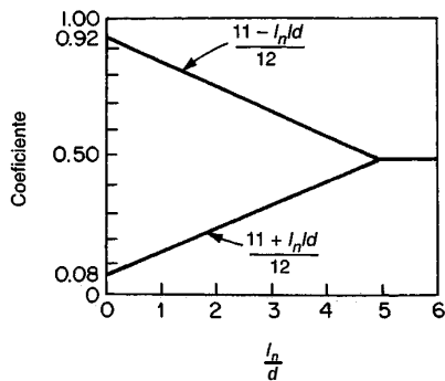
FIGURA 4.24 Coeficientes de efectividad para el refuerzo en el alma vertical y horizontal en vigas de gran altura.
