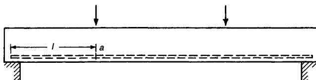
FIGURA 5.7 Longitud de desarrollo.
