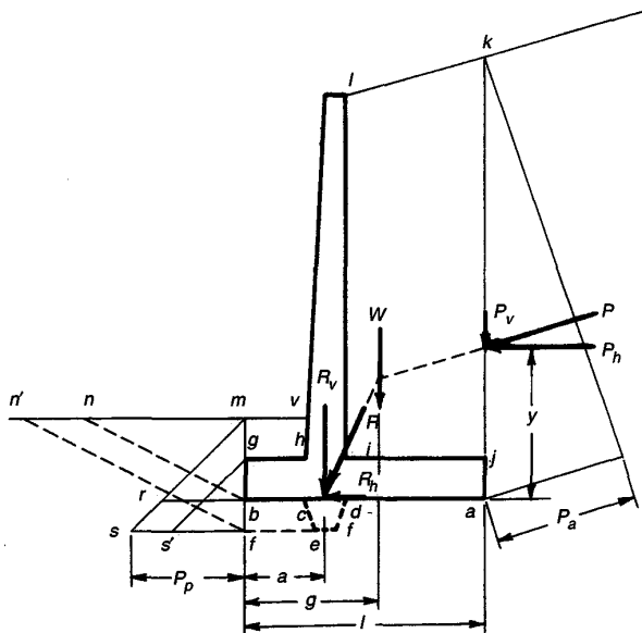
FIGURA 17.4 Estabilidad externa de un muro en voladizo.
