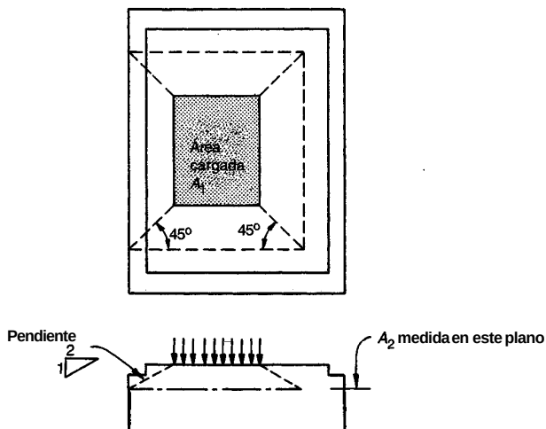
FIGURA 16.8 Definición de las áreas A_1 y A_2 .
