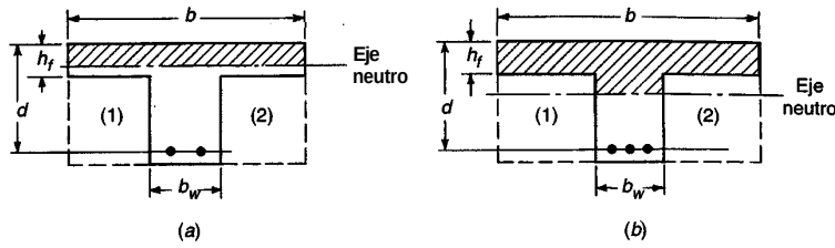
FIGURA 3.14 Secciones transversales efectivas para vigas T.
