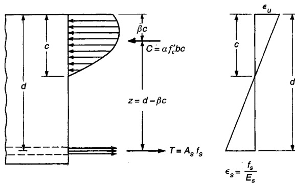
FIGURA 3.6 Distribución de esfuerzos para la carga última.
