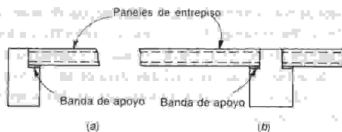
FIGURA 18.32 Conexiones de losa a viga.
