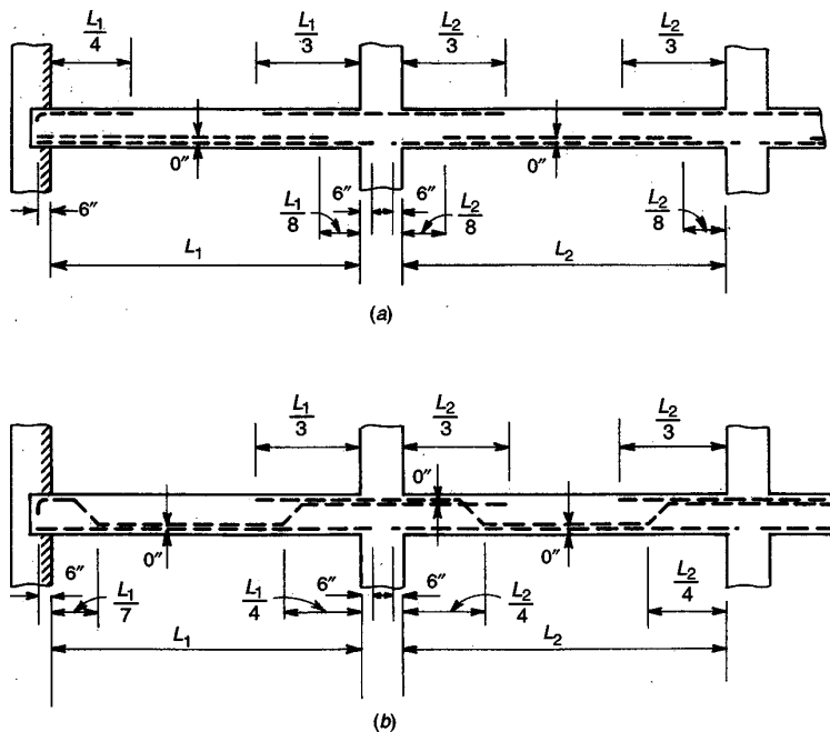
FIGURA 5.15 Puntos estándar de corte y doblamiento para barras en luces aproximadamente iguales con cargas distribuidas de manera uniforme.
