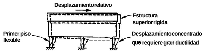
FIGURA 20.4 Primer piso blando que soporta una estructura superior más rígida.
