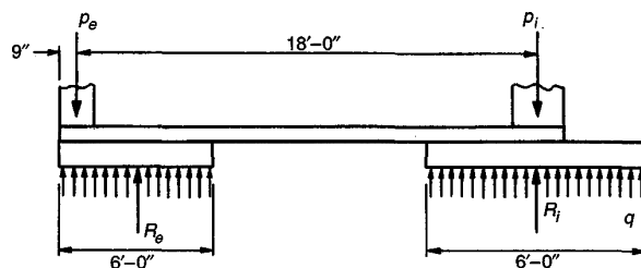
FIGURA 16.17 Fuerzas y reacciones en las zapatas con viga de amarre del ejemplo 16.4.
