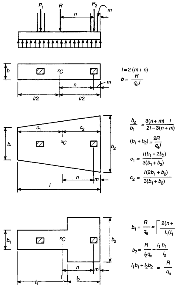
FIGURA 16.14 Zapatas para dos columnas (adaptada de la referencia 16.7).
