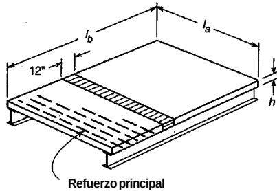
FIGURA 12.3 Principio básico de la franja unitaria para el diseño a flexión.
