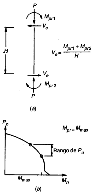
FIGURA 20.15 (a) Fuerzas consideradas en el diseño a cortante de columnas sometidas a carga sísmica, (b) diagrama de interacción usado para determinar la resistencia a momento máximo probable. Observe que M_{pr} de columnas usualmente es gobernado por M_{pr} de las vigas que llegan al nudo en vez de M_u .
