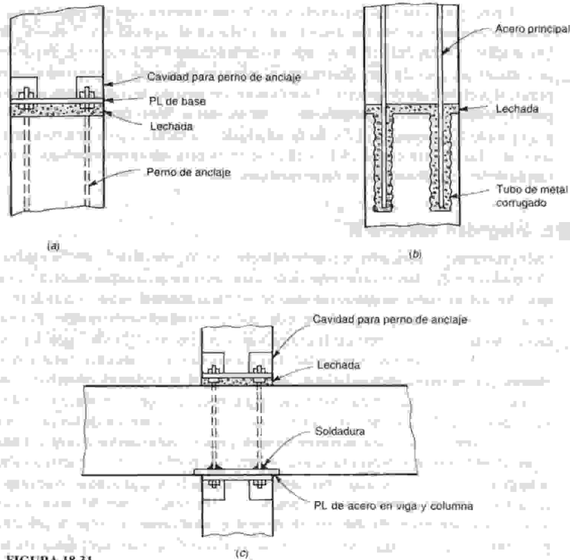
FIGURA 18.31 Conexiones de columna a columna.
