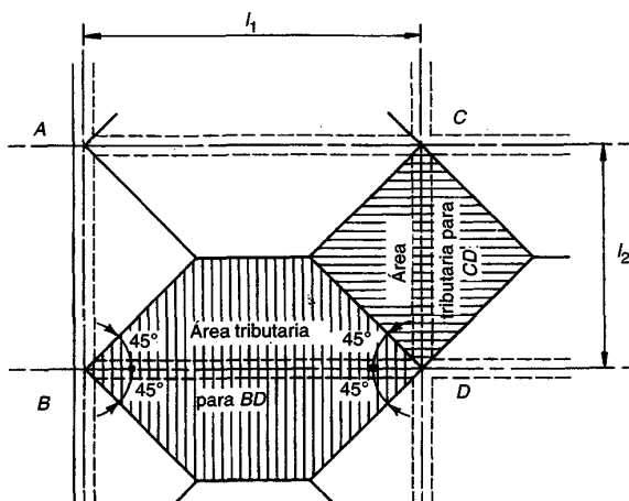
FIGURA 13.6 Áreas tributarias para cálculos de cortante.
