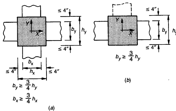
FIGURA 10.7 Confinamiento de nudos de concreto mediante vigas: (a) confinamiento en las direcciones X y Y; (b) confinamiento en la dirección X únicamente.
