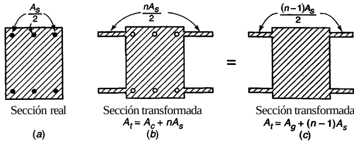
FIGURA 1.16 Sección transformada para compresión axial.
