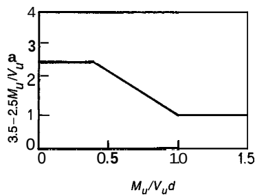
FIGURA 4.23 Multiplicador de la resistencia a cortante para vigas de gran altura.
