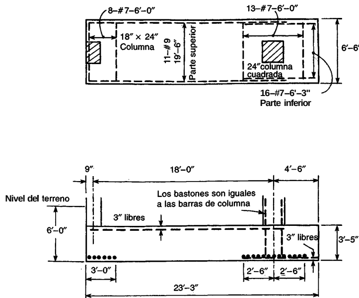
FIGURA 16.15 Zapata combinada del ejemplo 16.3.
