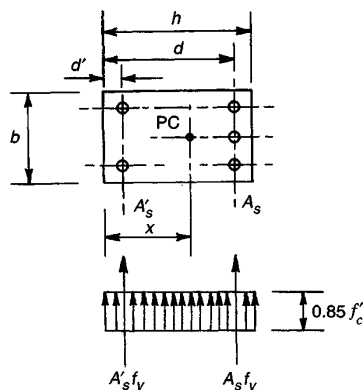
FIGURA 8.12 Centroide plástico de una columna reforzada asimétricamente.
