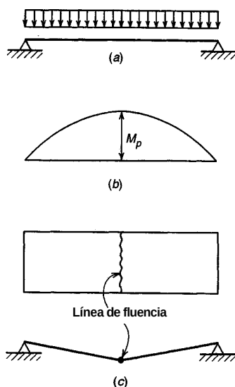
FIGURA 14.1 Losa armada en una dirección, simplemente apoyada y cargada de manera uniforme.
