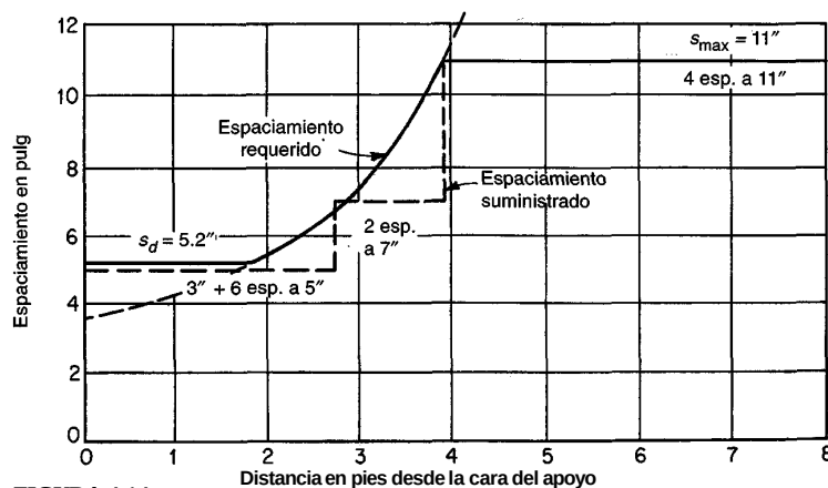
FIGURA 4.14 Espaciamientos requeridos para los estribos del ejemplo 4.3.
