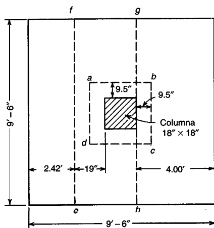
FIGURA 16.10 Secciones críticas para el ejemplo 16.2.
