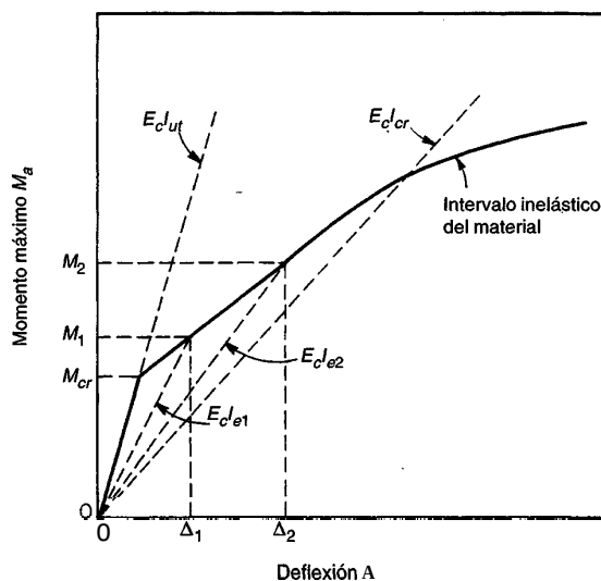
FIGURA 6.5 Deflexión de una viga de concreto reforzado.
