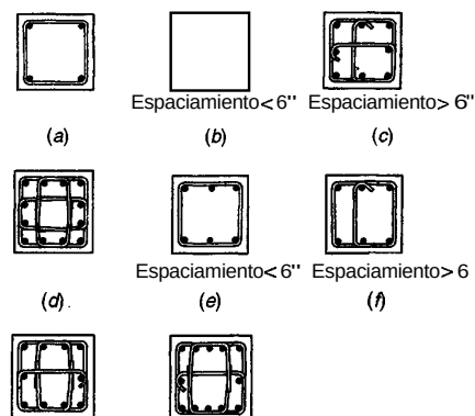
FIGURA 8.2 Distribución de flejes en columnas cuadradas y rectangulares.
