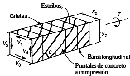
FIGURAS 7.7 Analogía de armadura espacial.
