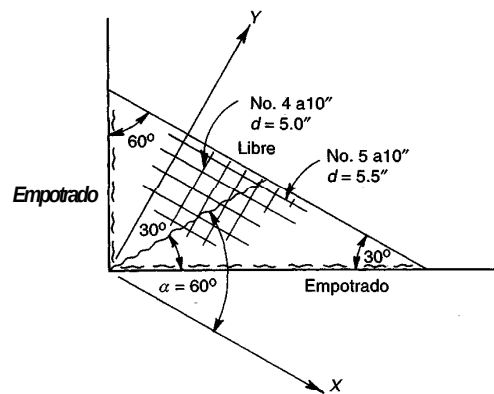
FIGURA 14.12 Ejemplo de línea de fluencia oblicua.
