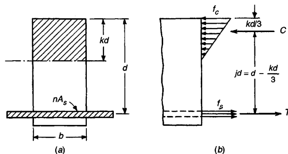
FIGURA 3.5 Sección transformada y fisurada.
