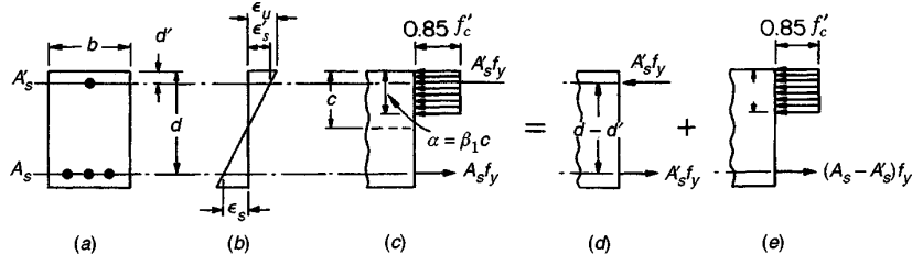
FIGURA 3.11 Viga rectangular doblemente reforzada.
