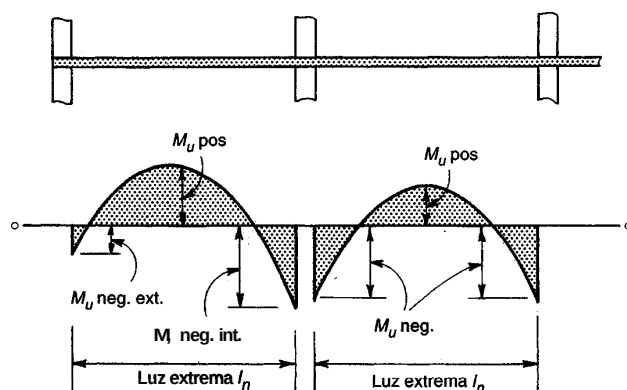
FIGURA 13.4 Distribución del momento estático total M_o a las secciones críticas para flexión positiva y negativa.
