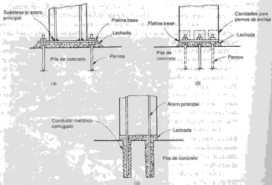
FIGURA 18.28 Conexiones para la base de columnas.
