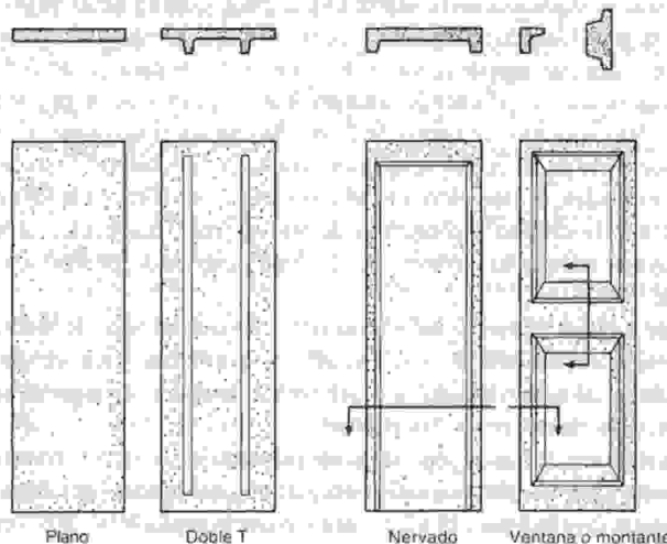
FIGURA 18.15 Paneles de muro en concreto prefabricado.
