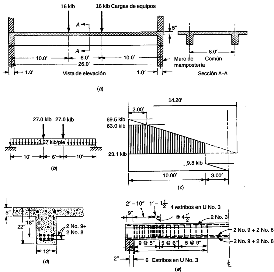
FIGURA 5.17 Ejemplo de diseño de una viga T.
