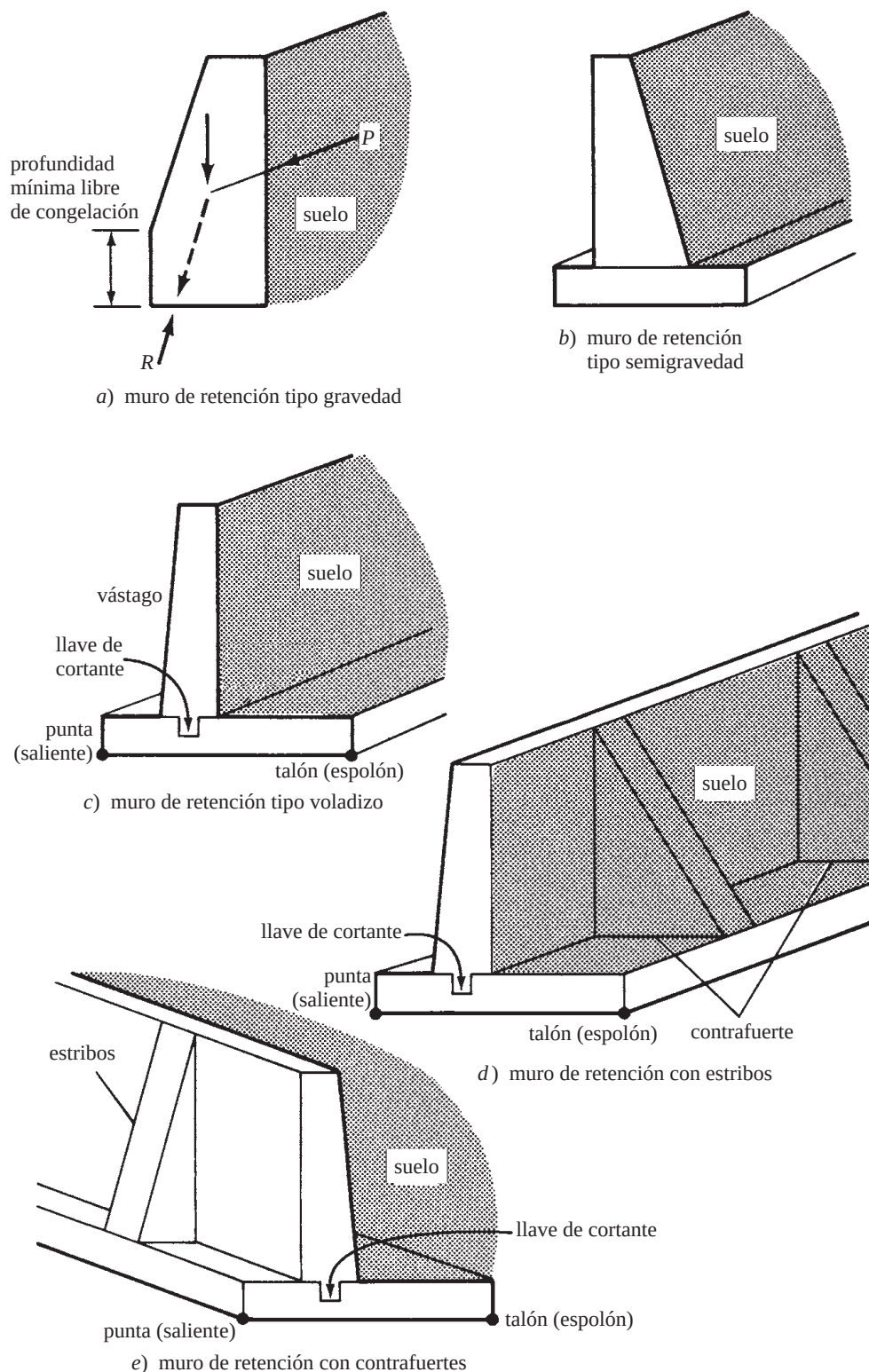
Figura 13.1 Muros de retención.
