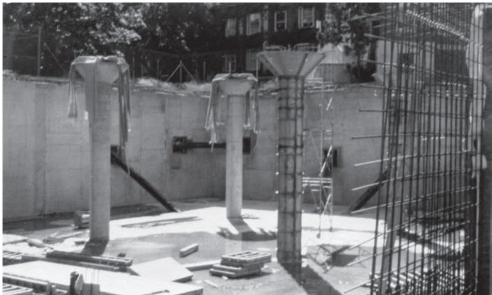
Columnas redondas. (Cortesía de Economy Forms Corporation.)
