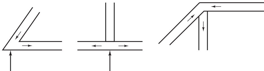
Figura C.7 Diferentes tipos de nodos de armadura.
