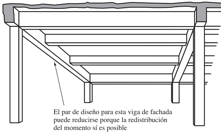
Figura 15.7 Torsión de compatibilidad.
