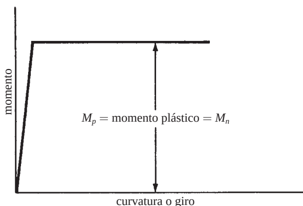
Figura 14.4 Relación momento-curvatura de un material plástico ideal.
