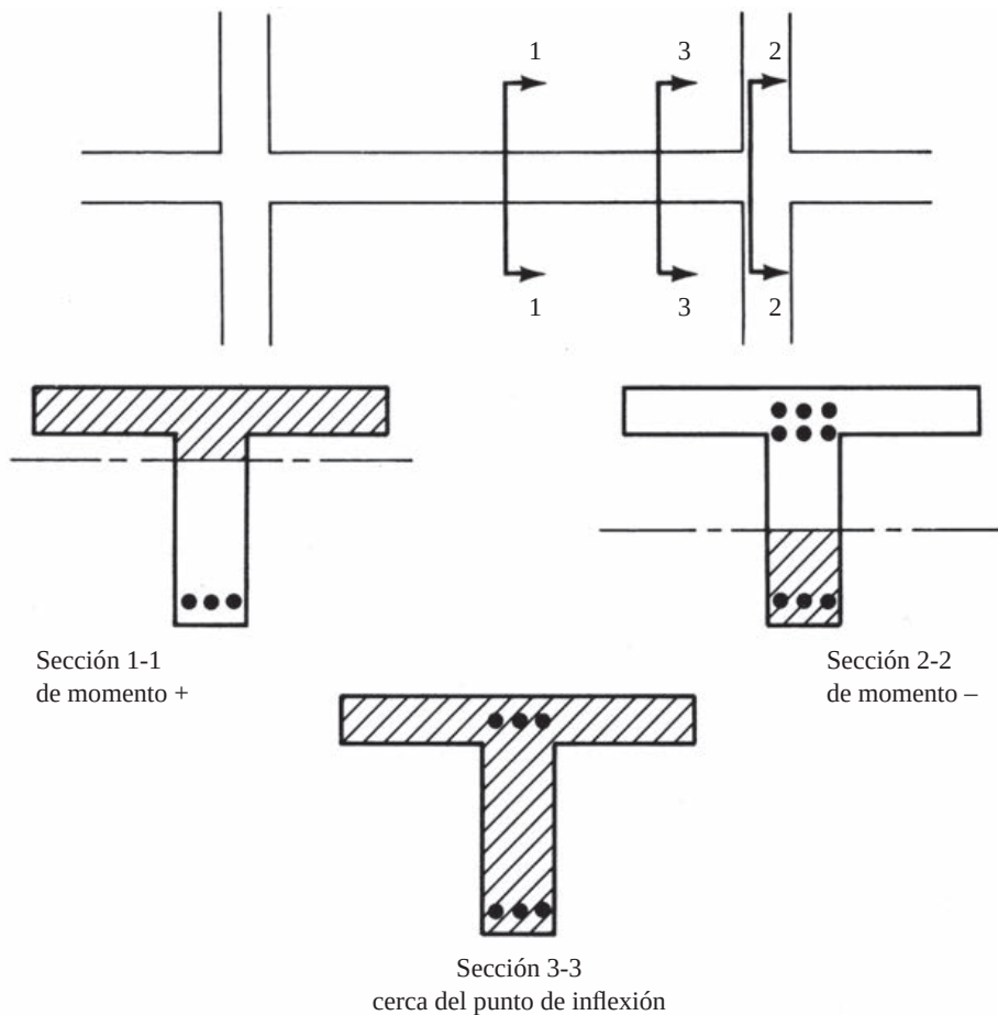
Figura 6.6 Deflexiones en una viga T continua.
