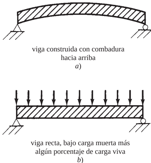
Figura 6.1 Combadura (o contraflecha).
