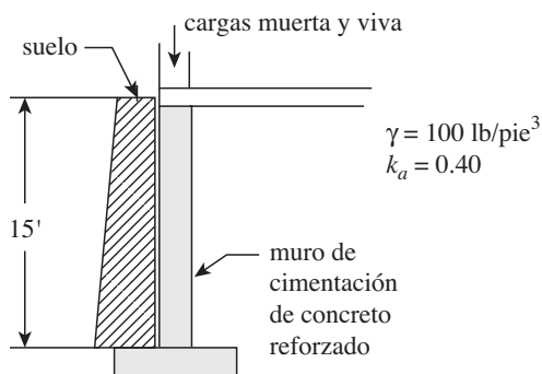
Figura 18.2 Muro de cimentación.
