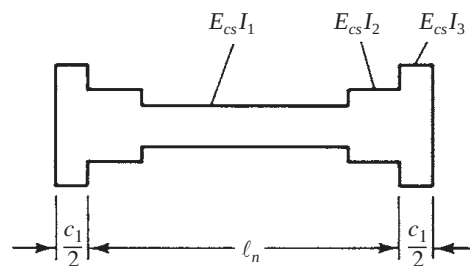
e) diagrama de rigidez de viga losa equivalente
