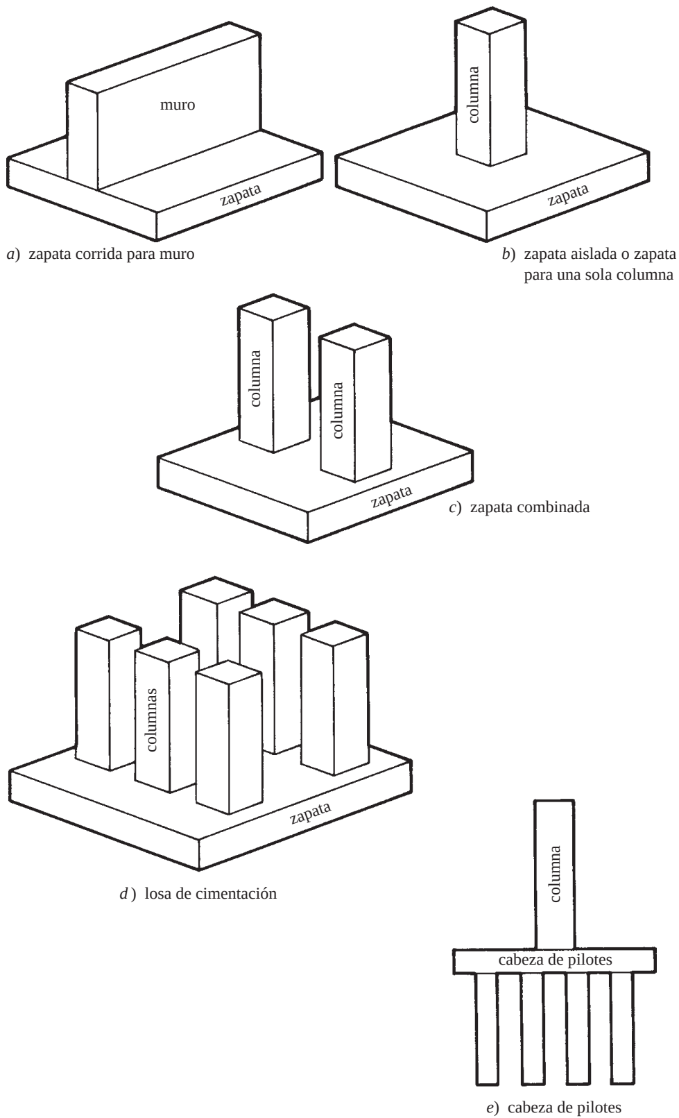
Figura 12.1 Tipos de zapatas.
