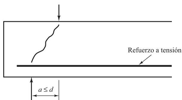
Figura C.3 Un claro de cortante muy corto.
