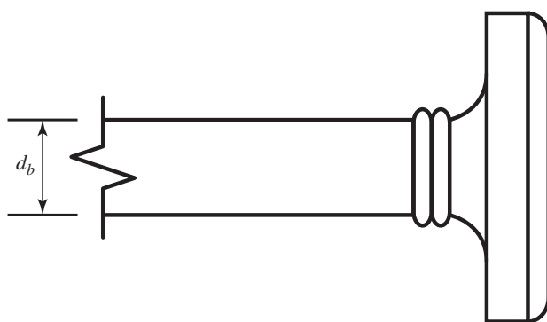
Figura 1.3 Varilla de refuerzo corrugada con anclaje interno.
