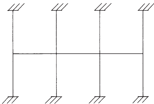
Figura 16.2 Método del marco equivalente.
