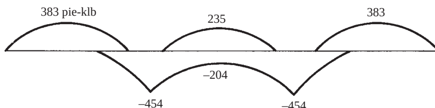
Figura 14.18 Envolvente de momentos.
