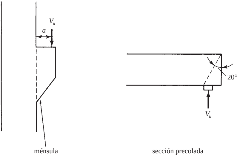
Figura 8.19 Fallas posibles por fricción al cortante.
