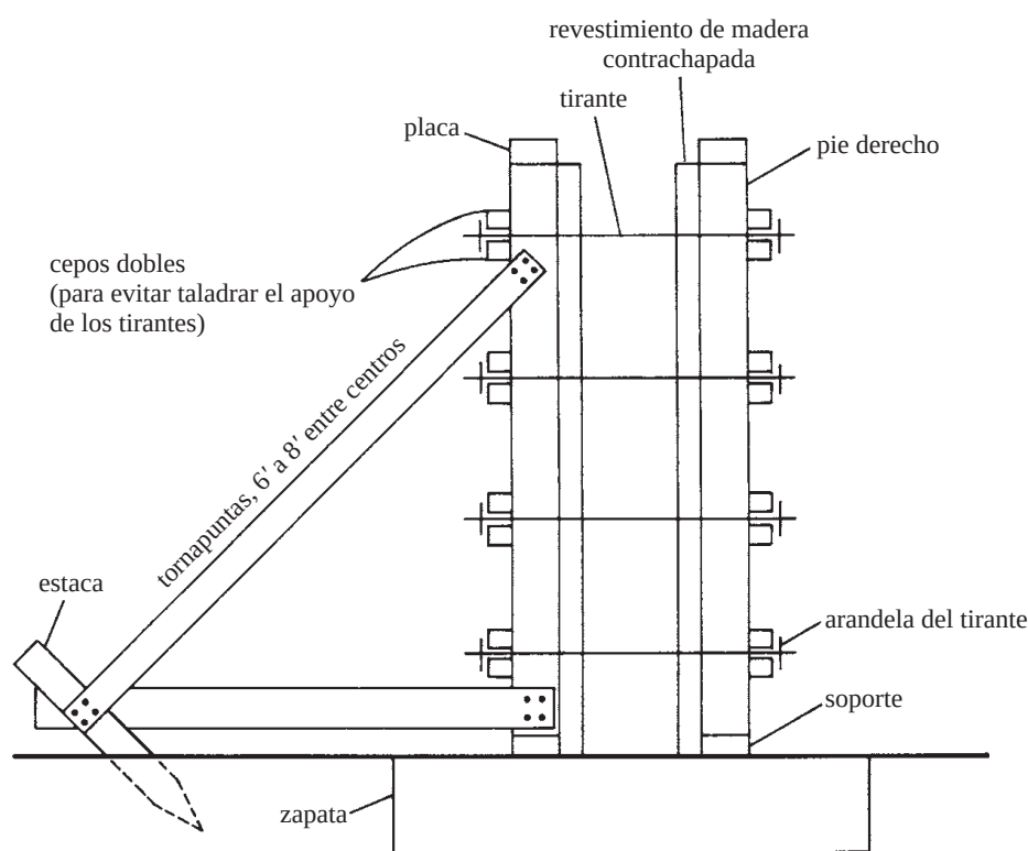
Figura 20.2 Cimbra de madera para un muro.
