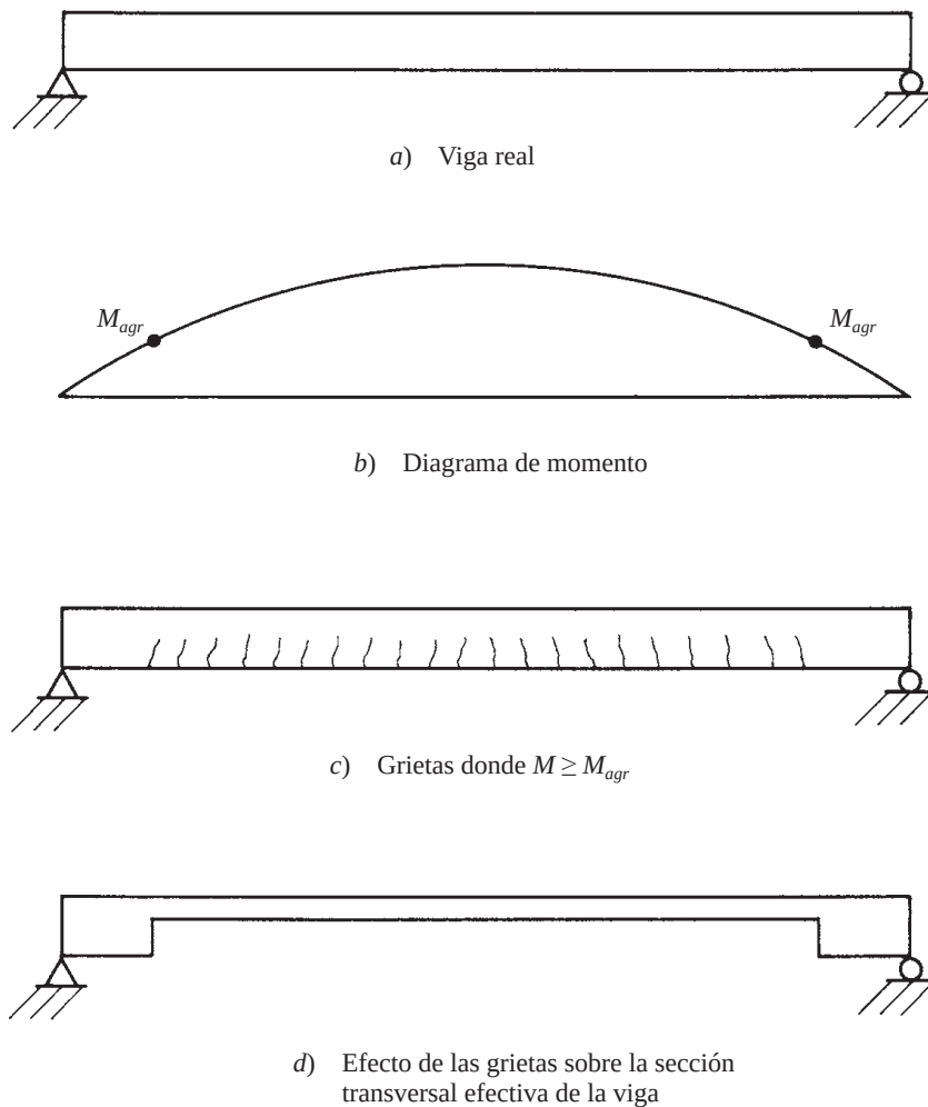
Figura 6.3 Efectos de las grietas en las deflexiones.
