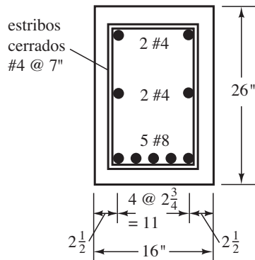
Figura 15.14 Refuerzo seleccionado para la viga del ejemplo 15.1.
