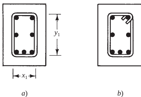
Figura 15.3 Estribos cerrados (éstos son frecuentemente imprácticos).
