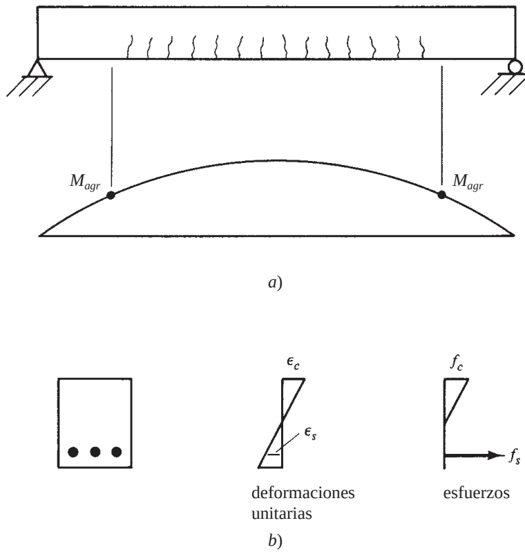
Figura 2.2 Concreto agrietado: etapa de esfuerzos elásticos.
