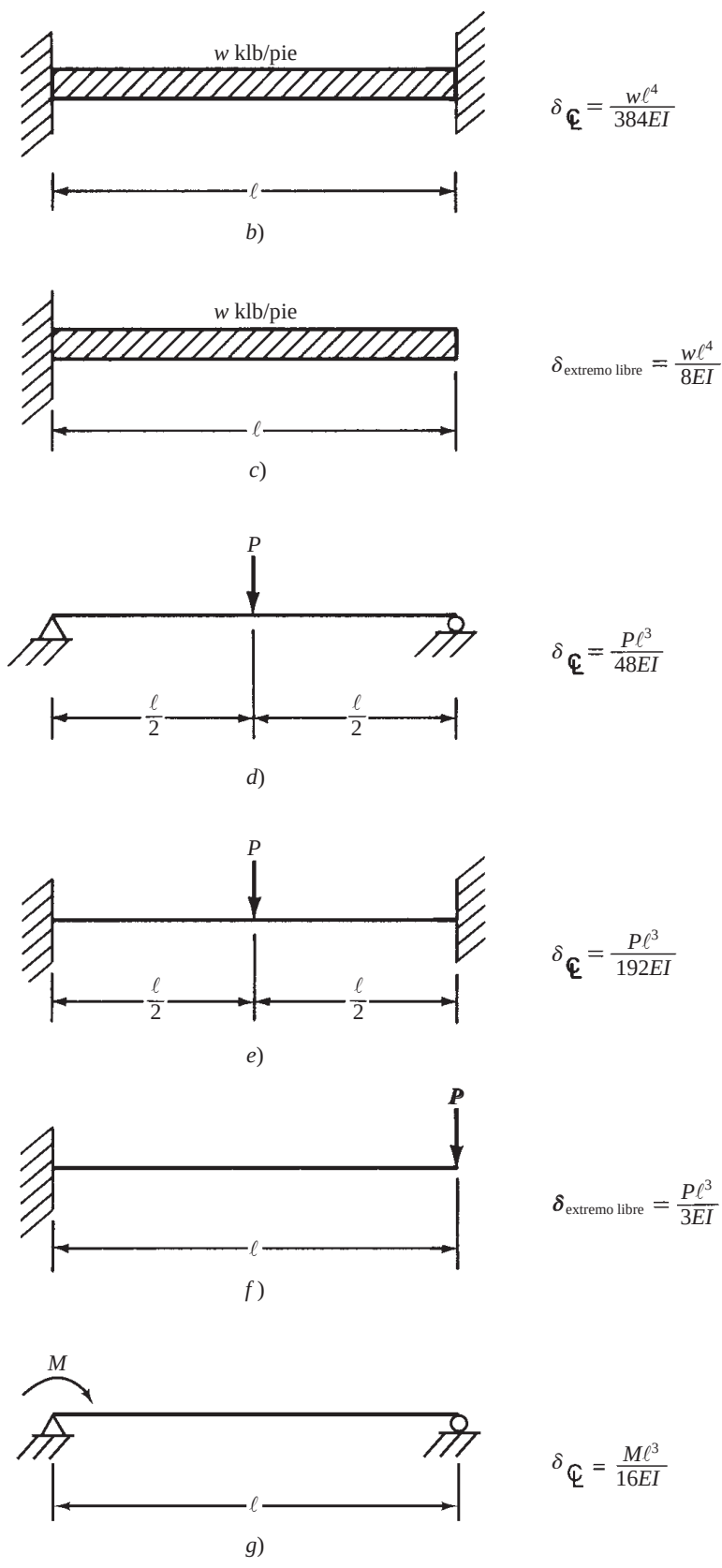
Figura 6.2b-g) Expresiones para algunas deflexiones.
