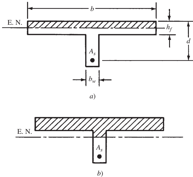
Figura 5.2 Posiciones del eje neutro.
