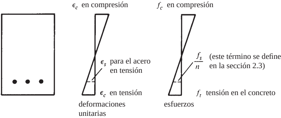
Figura 2.1 Etapa del concreto no agrietado.
