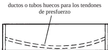
Figura 19.4 Viga postensada.
