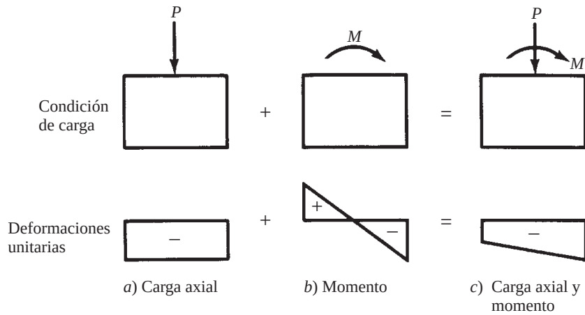
Figura 10.3 Deformaciones unitarias en la columna.
