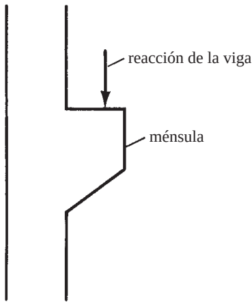
Figura 8.9 Ménsula que soporta reacción de viga.
