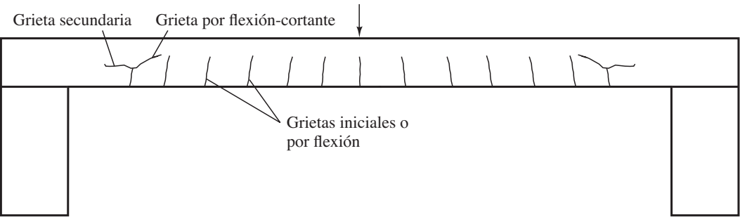
Figura 8.1 Grietas por flexión-cortante.
