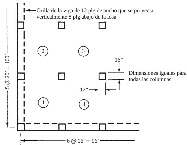
Figura 16.6 Una losa de piso de placa plana.
