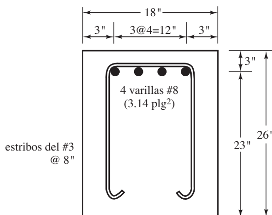
Figura 7.10 Sección transversal de viga en voladizo.
