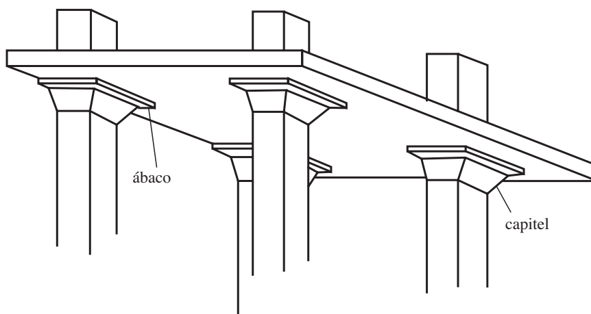
c) losa plana
