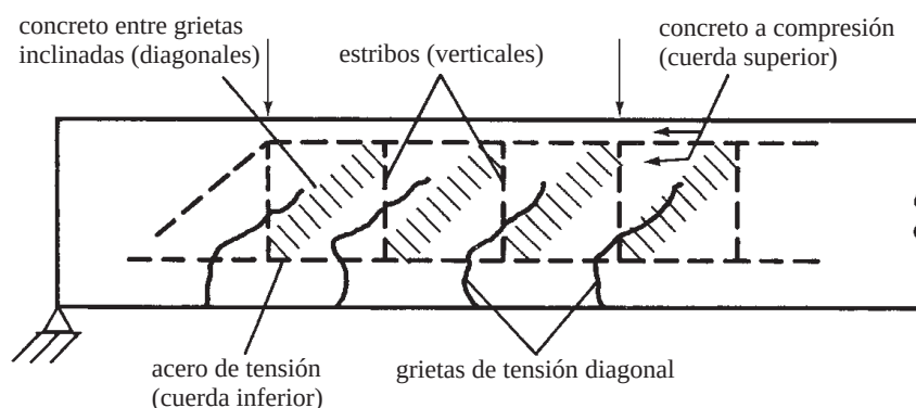
Figura 8.4 Analogía de la armadura.
