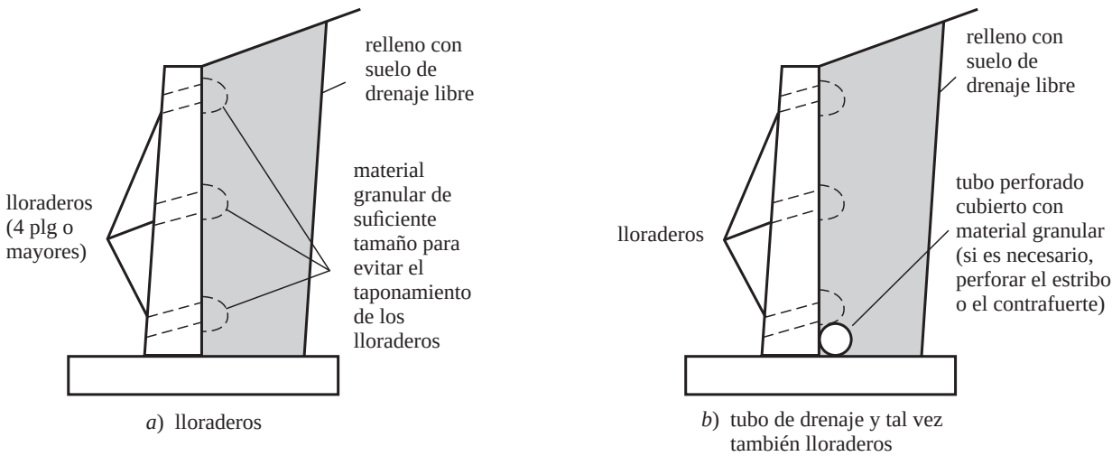
Figura 13.3 Drenaje de un muro de retención.
