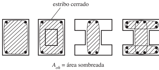
Figura 15.12 Valores de A_{oh} .
