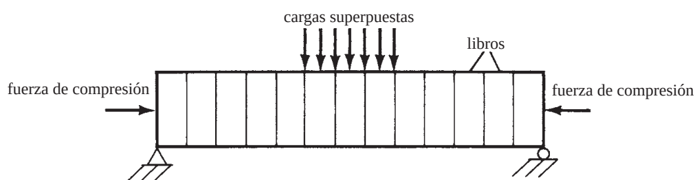
Figura 19.1 Presfuerzo.
