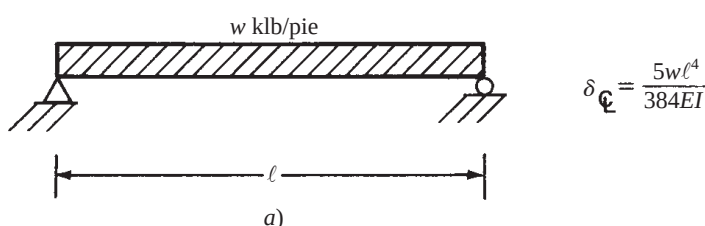
Figura 6.2a) Expresiones para algunas deflexiones.
