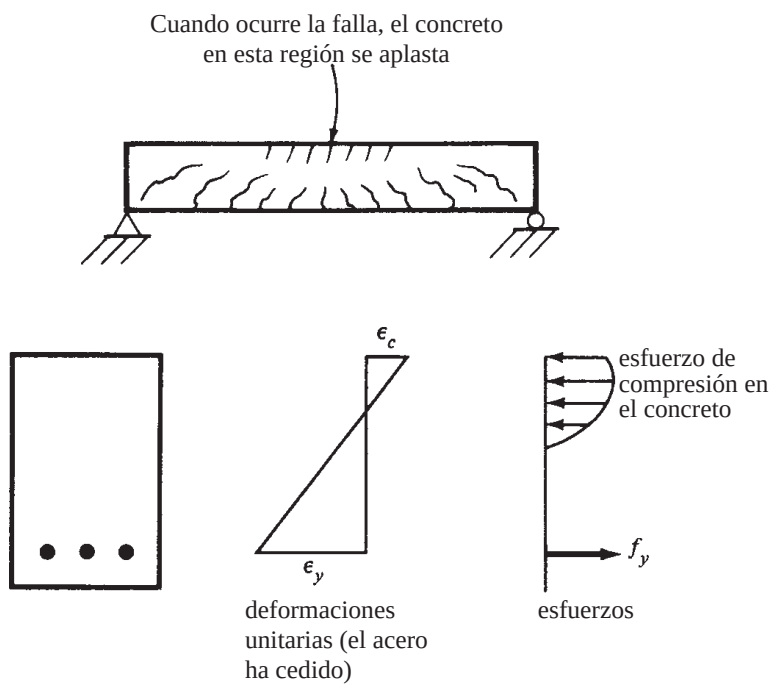
Figura 2.3 La etapa de resistencia última.
