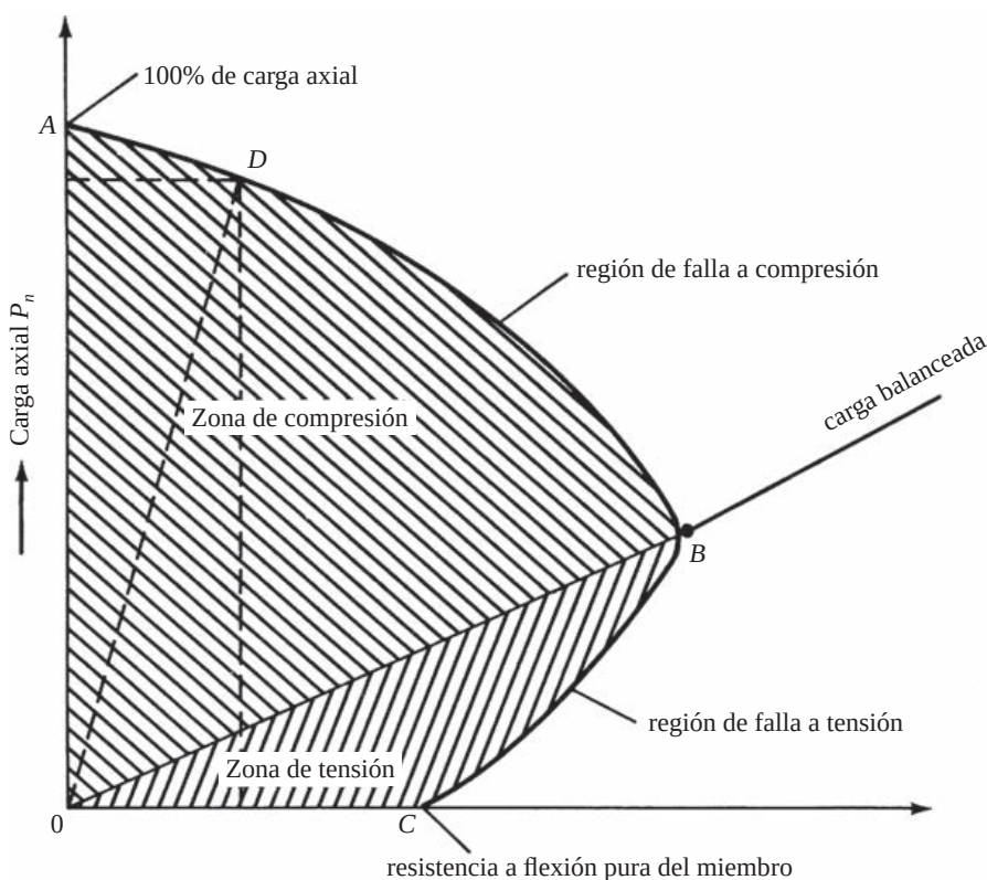
Figura 10.10 Diagrama de interacción de columna.
