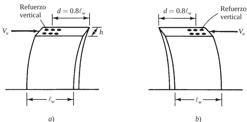
Figura 18.6 Muro de cortante.
