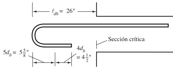
Figura 7.16 Gancho de 180°.
