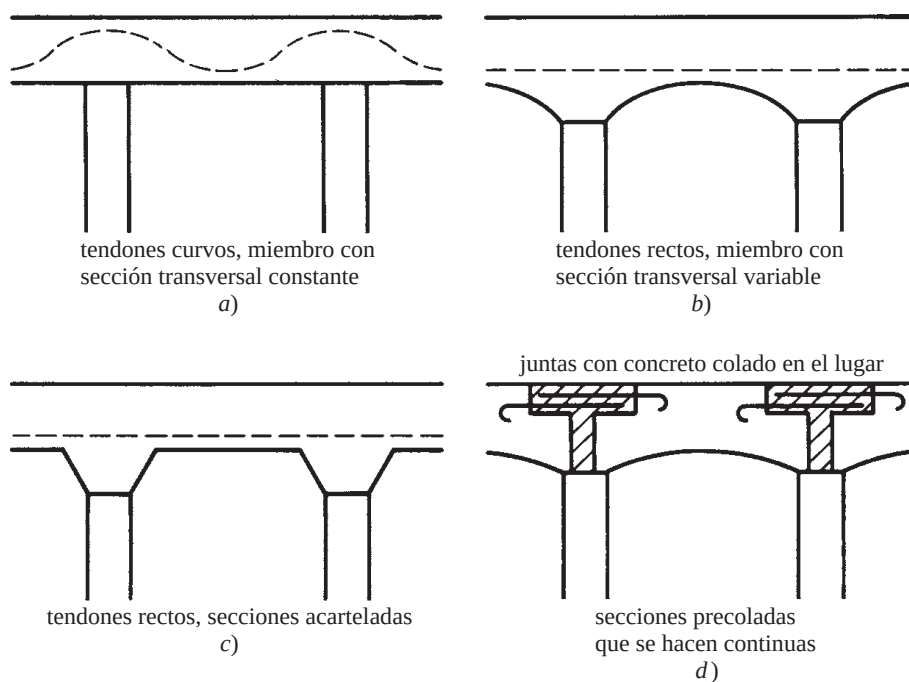
Figura 19.14 Vigas continuas.
