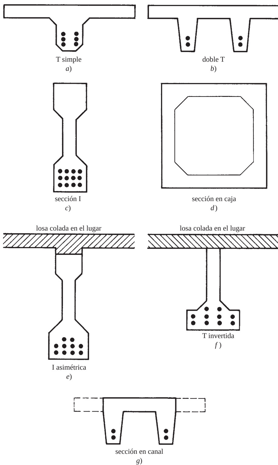
Figura 19.8 secciones presforzadas comúnmente aplicadas.
