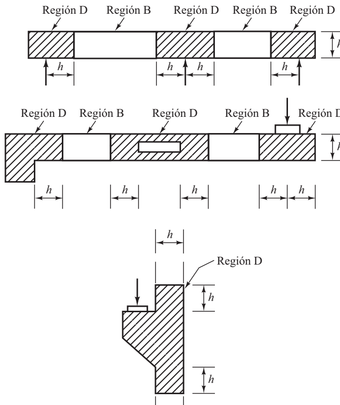
Figura C.2 Regiones B y D.
