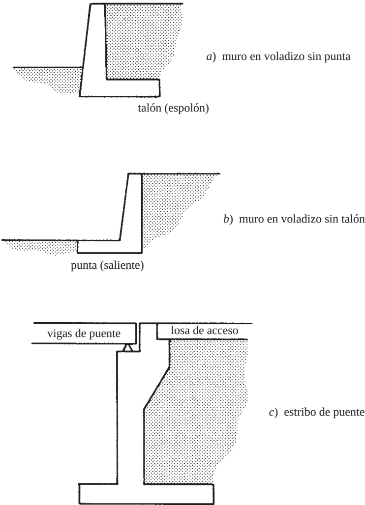
Figura 13.2 Otros tipos de muros de retención.
