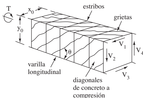
Figura 15.10 Armadura espacial imaginaria.
