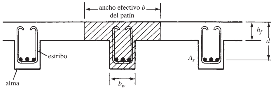
Figura 5.1 Ancho efectivo de vigas T.
