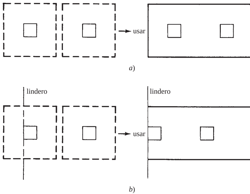
Figura 12.18 Uso de zapatas combinadas.
