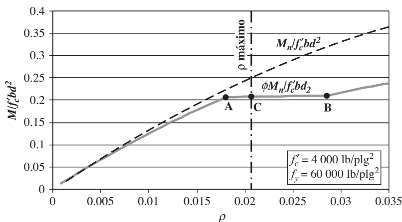
Figura 3.6 Capacidad de momento contra \rho .
