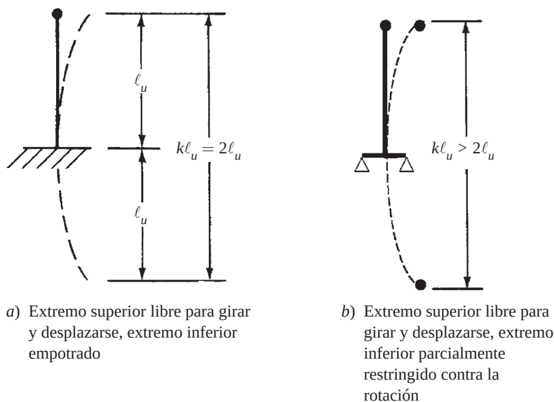
Figura 11.2 Columnas para marcos no riostrados.
