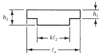
b) sección 2-2
