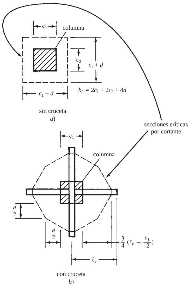
Figura 16.5 Secciones críticas por cortante.
