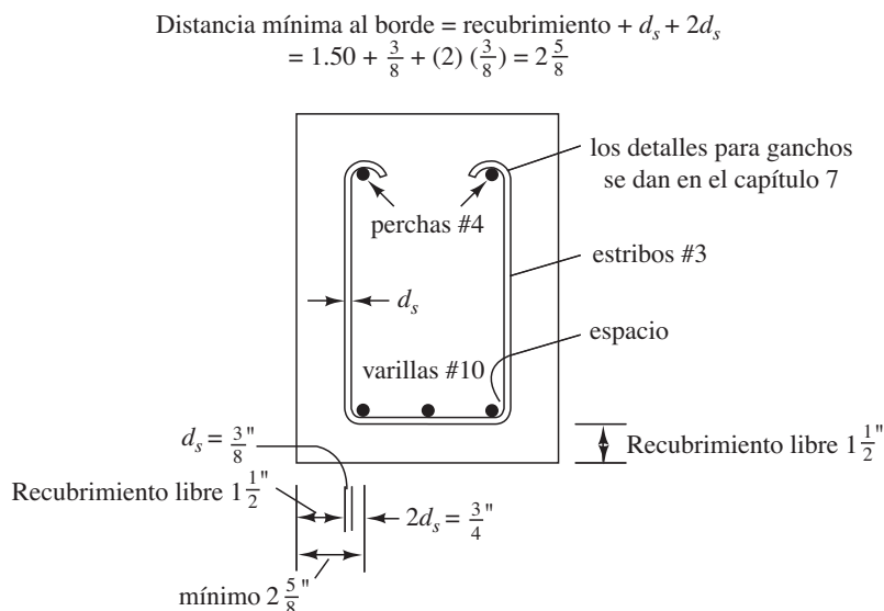
Figura 4.1 Determinación de la distancia mínima al borde.
