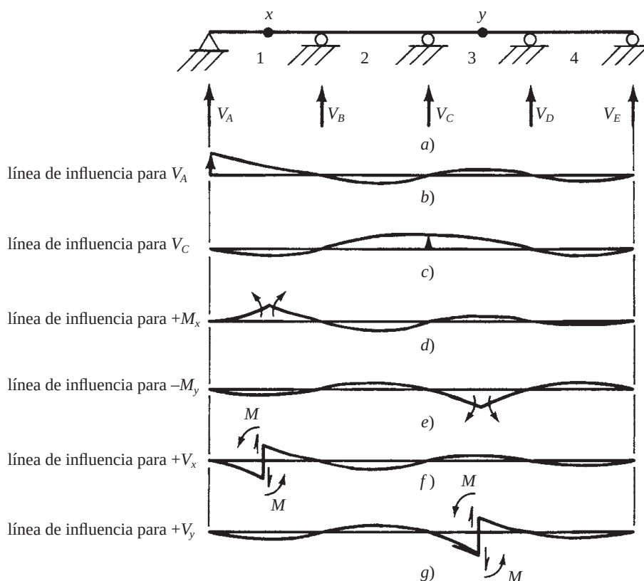
Figura 14.1 Líneas de influencia cualitativas.
