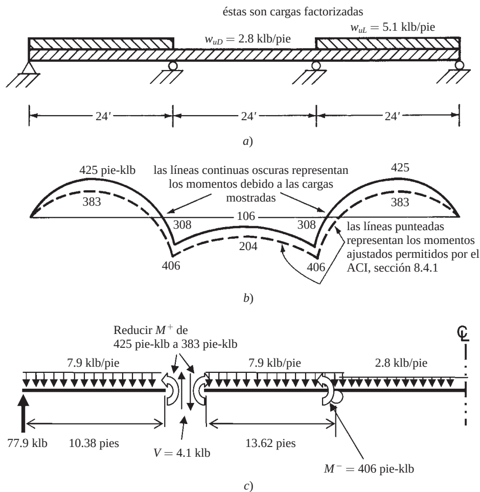
Figura 14.15 Momento positivo máximo en los claros extremos. a) Patrones de carga para el momento positivo máximo en ambos claros extremos. b) Diagrama de momentos antes y después de reducir el momento positivo en los claros extremos. c) Fuerzas cortantes y momentos en el claro izquierdo después de reducir M^+ 10% en los claros extremos.
