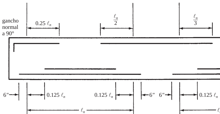
Figura 14.37 Detalles recomendados en varillas de vigas continuas.
