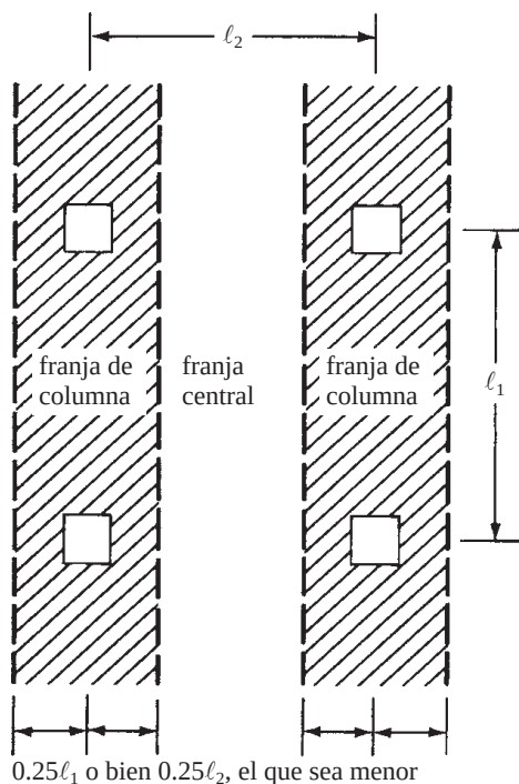
Figura 16.3 Franjas de columna y central.
