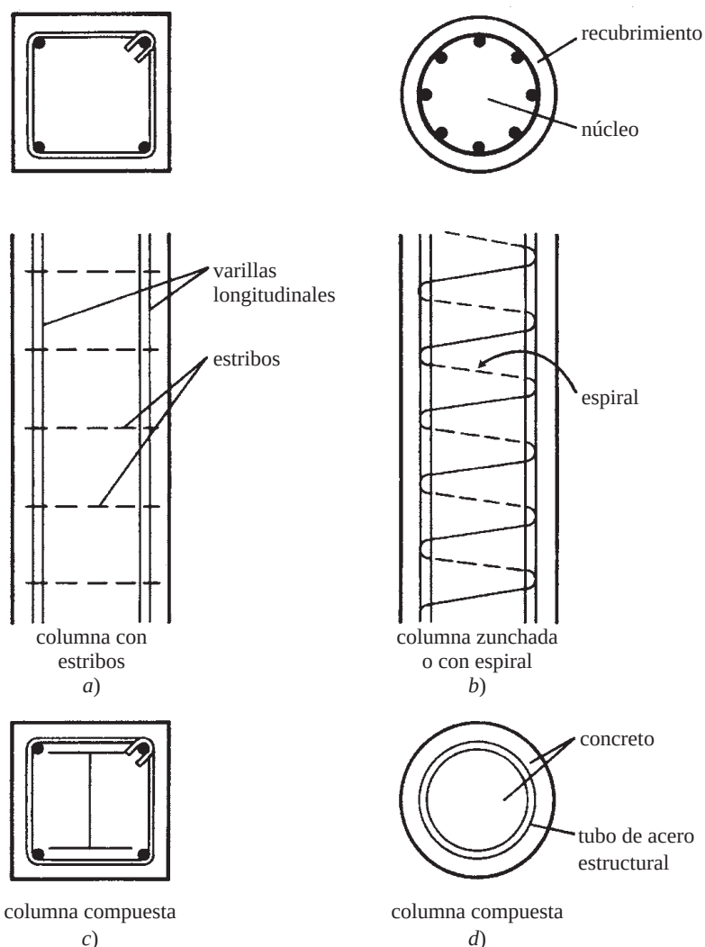
Figura 9.2 Tipos de columnas.
