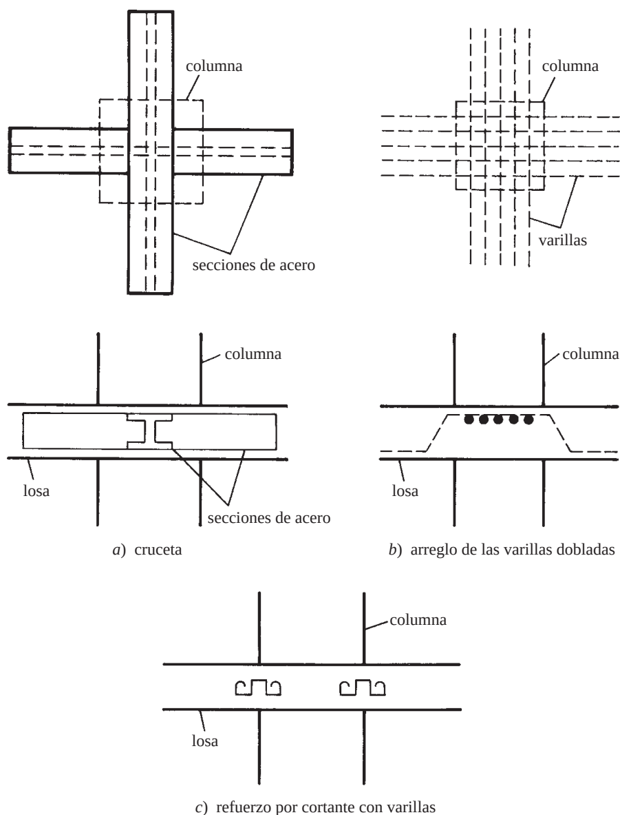
Figura 16.4 Refuerzo por cortante en losas y columnas.
