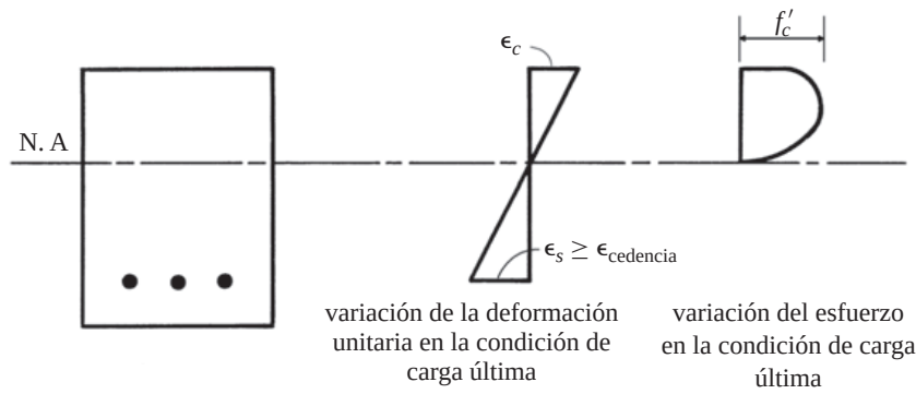
Figura 3.1 Carga última.
