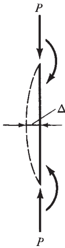
Figura 11.5 Amplificación de momentos en una columna sin desplazamiento lateral.
