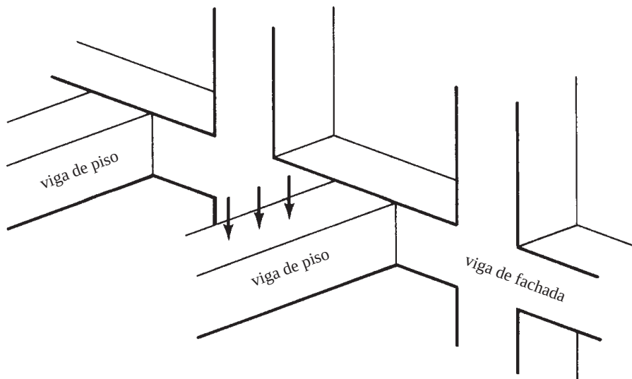
Figura 15.1 Torsión en vigas de fachada.
