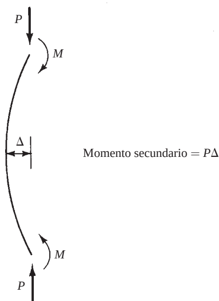
Figura 9.1 Momento secundario o momento P\Delta .
