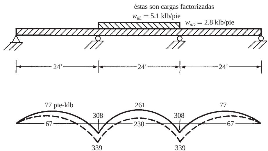
Figura 14.16 Momento positivo máximo en el claro 2.
