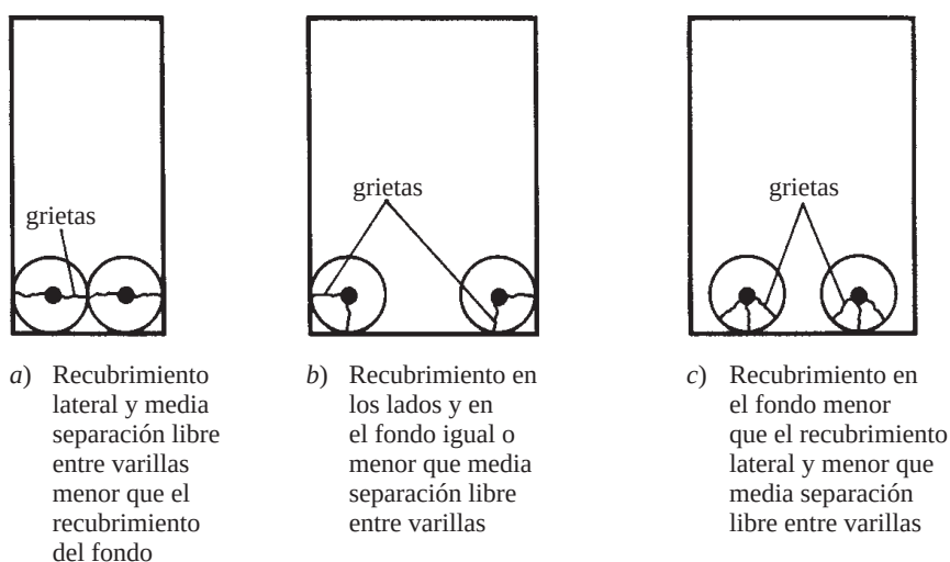
Figura 7.6 Tipos de falla por adherencia.
