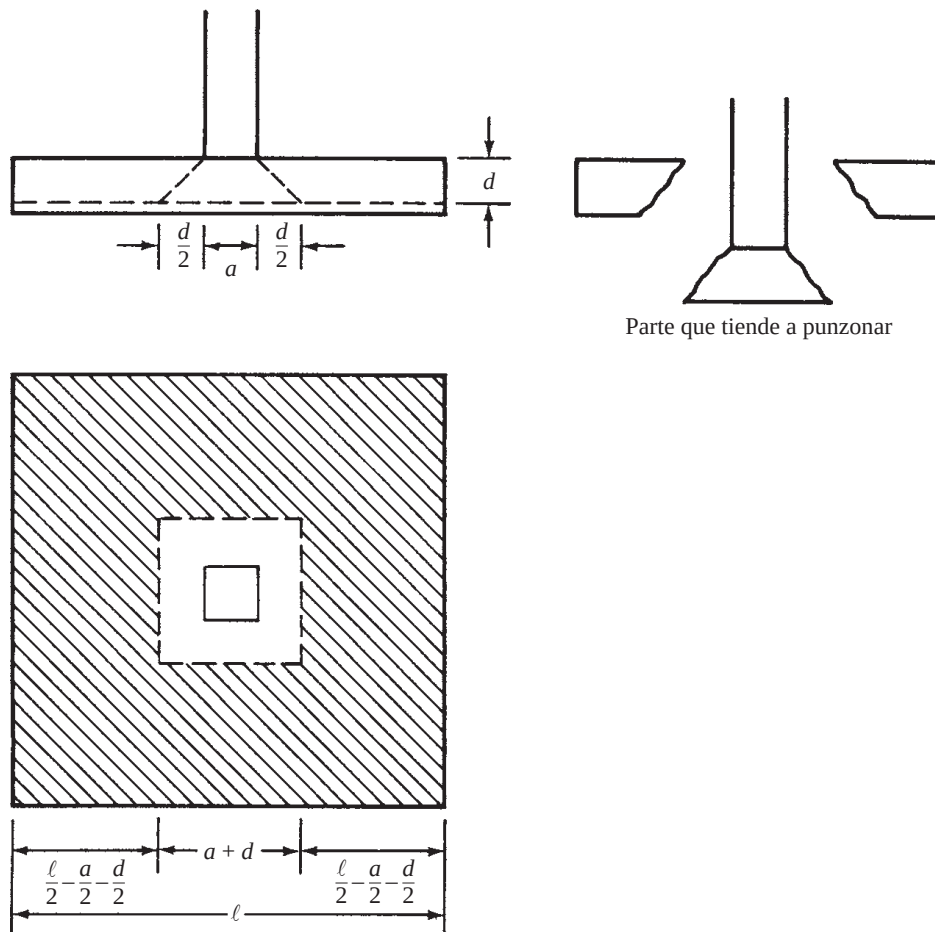
Figura 12.9 Cortante en dos direcciones o por perforación.
