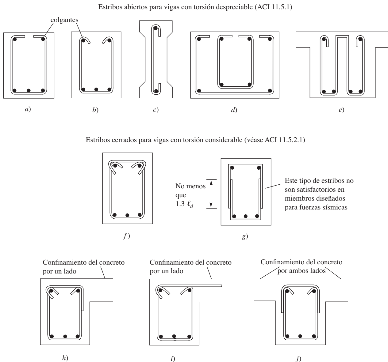
Figura 8.3 Tipos de estribos.
