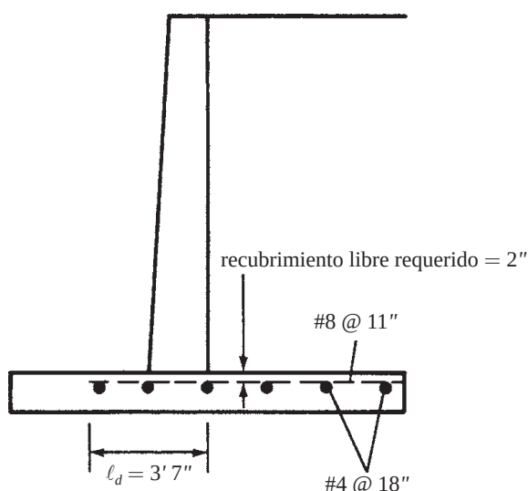
Figura 13.25 Refuerzo del talón.
