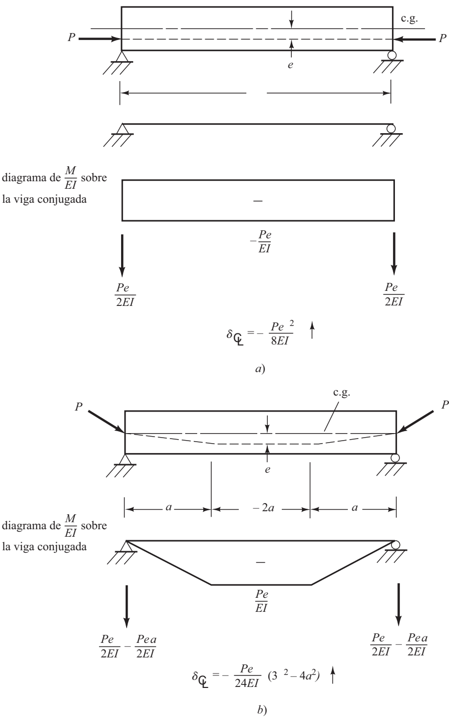
Figura 19.11 Deflexiones en vigas presforzadas. (Continúa.)
