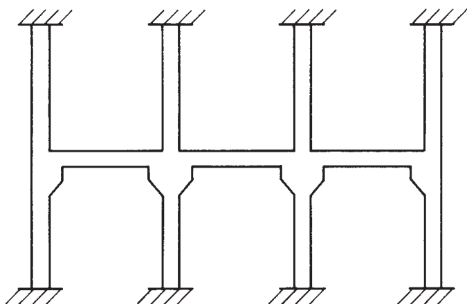
Figura 17.4 Marco equivalente para la franja sombreada de la figura 17.3 por carga vertical.
