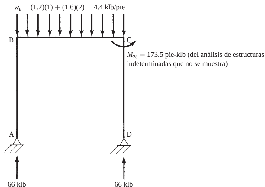
Figura 11.10 Carga 1.2D + 1.6L .
