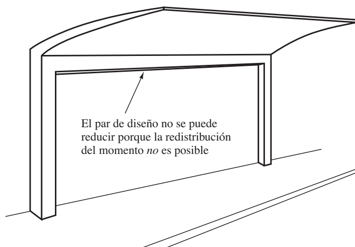
Figura 15.6 Torsión de equilibrio.
