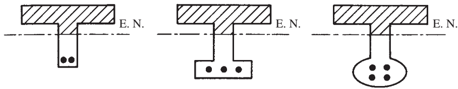
Figura 5.3 Diversas secciones transversales de vigas T.
