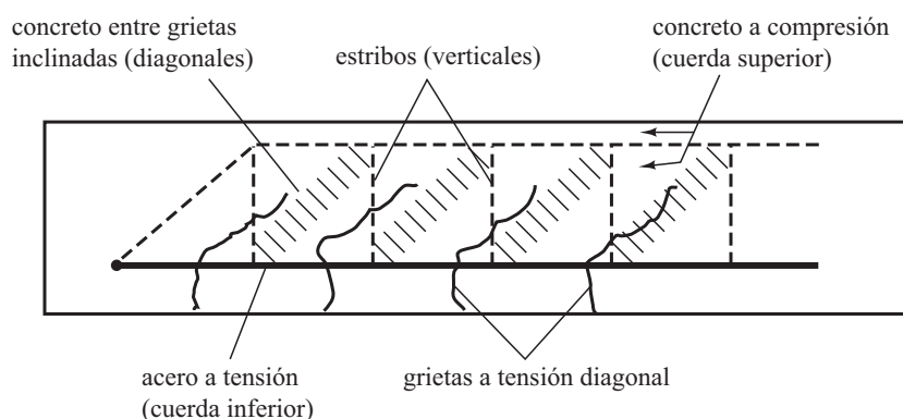
Figura C.4 Analogía de la armadura.
