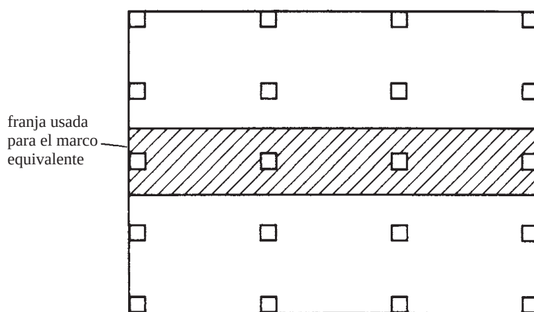
Figura 17.3 Viga de losa.
