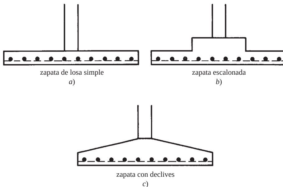
Figura 12.7 Formas de zapatas aisladas.
