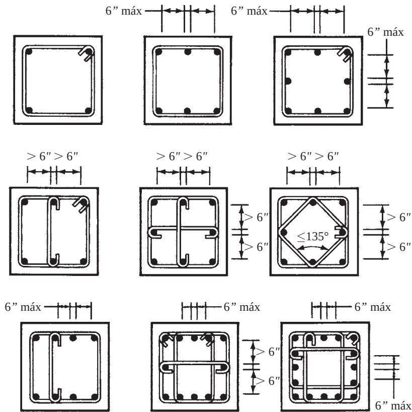
Figura 9.4 Disposiciones típicas de estribos.
