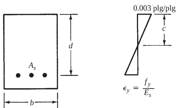
Figura 3.7 Condiciones balanceadas.
