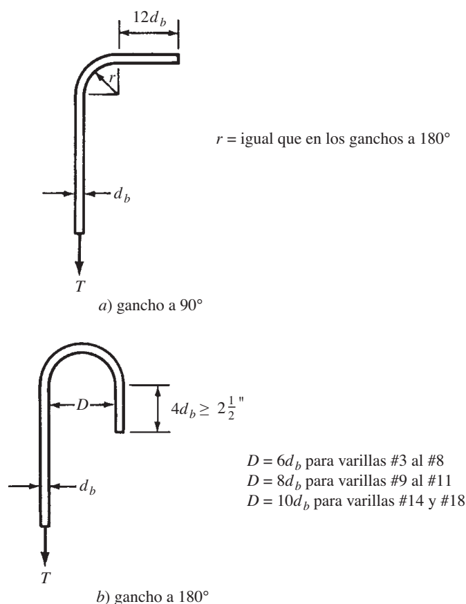
Figura 7.12 Ganchos.
