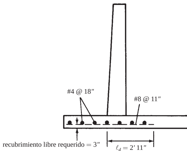
Figura 13.27 Refuerzo de la punta.
