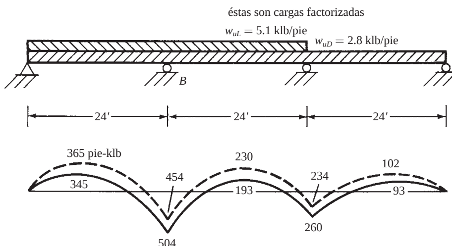
Figura 14.17 Momento negativo máximo en el apoyo B.
