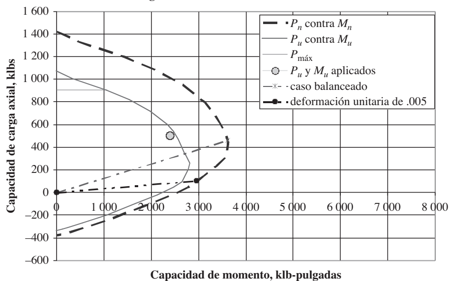
Diagrama de interacción de columna circular
