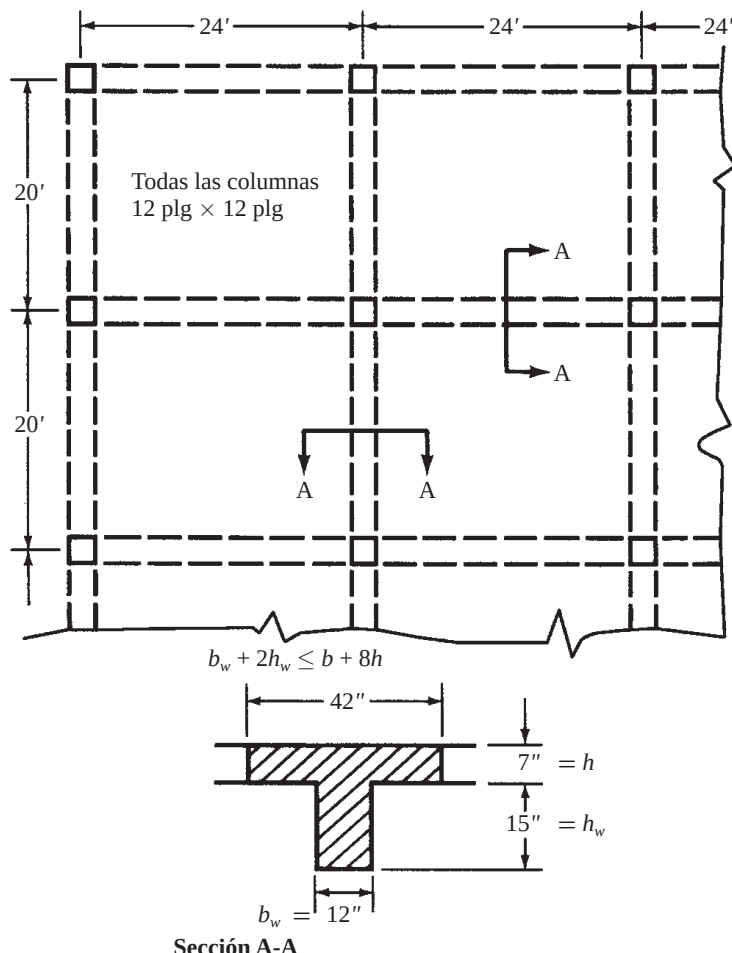
Figura 16.8 Losa en dos direcciones.
