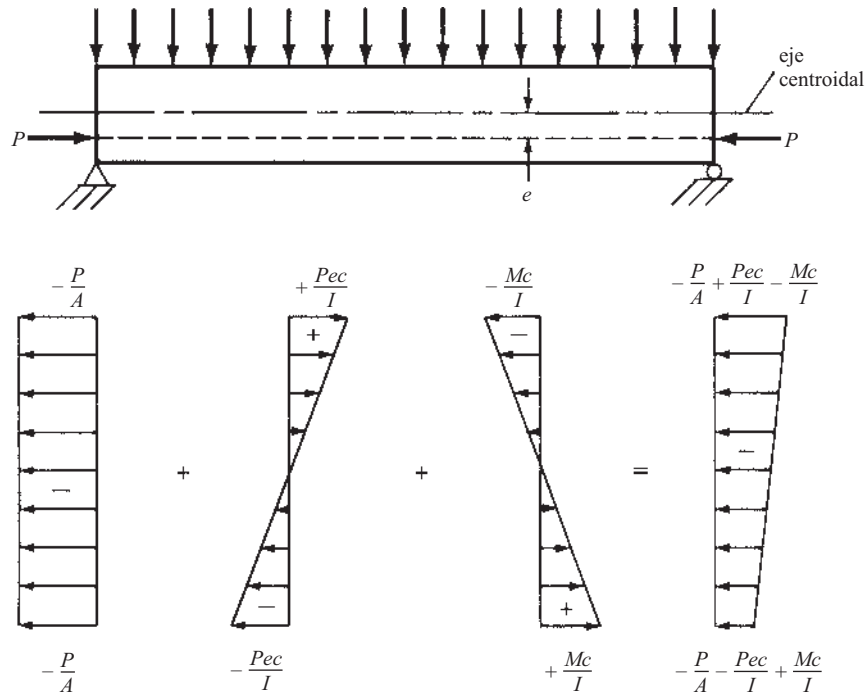
Figura 19.5 Distribución de esfuerzos en el concreto provenientes de la fuerza de presfuerzo excéntrica y de las cargas sobrepuestas.
