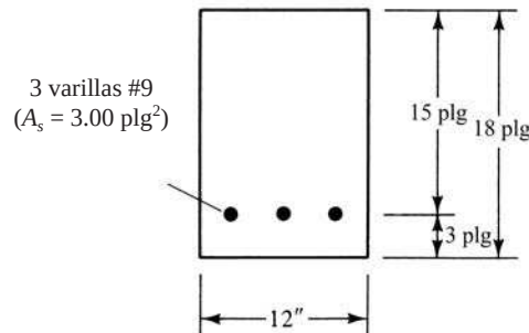
Figura 2.5 Sección transversal de la viga del Ejemplo 2.1.
