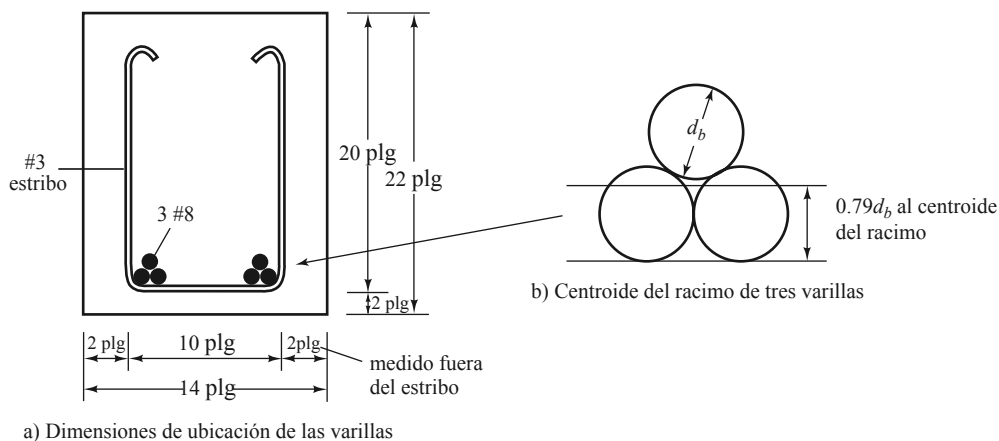
Figura 7.11 Sección transversal de la viga del Ejemplo 7.5.
