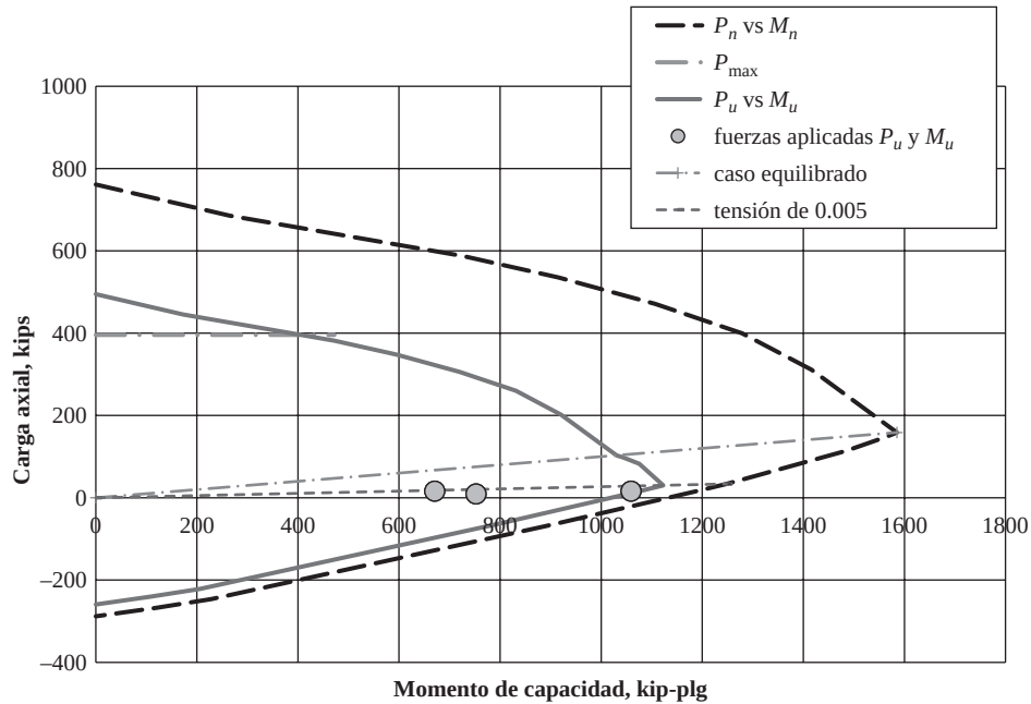
Figura 11.14 Diagrama de interacción para el Ejemplo 11.5: 12 plg \times 12 plg con A_{si} = 4.80 \text{ plg}^2 .
