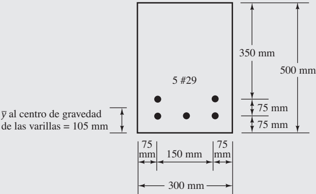
Figura 6.14 Sección transversal de la viga del Ejemplo 6.4.
