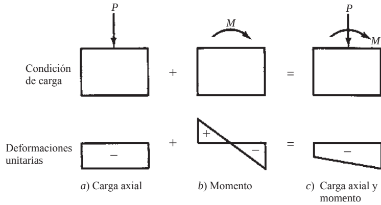
Figura 10.3 Deformaciones unitarias en la columna.
