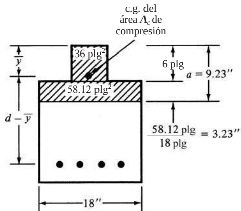
Figura 2.14 Área sujeta al bloque del esfuerzo de compresión del Ejemplo 2.9.
