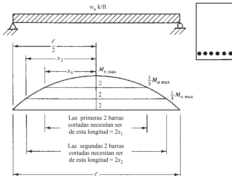
Figura 7.1 Ubicaciones teóricas de corte para una viga de un solo claro.
