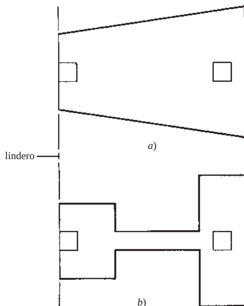
Figura 12.19 Zapatas trapezoidales y zapatas de tira o en forma de T.
