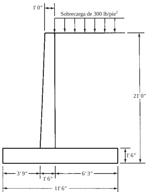
Figura 13.22 Dimensiones de un muro de retención para el Ejemplo 13.3.
