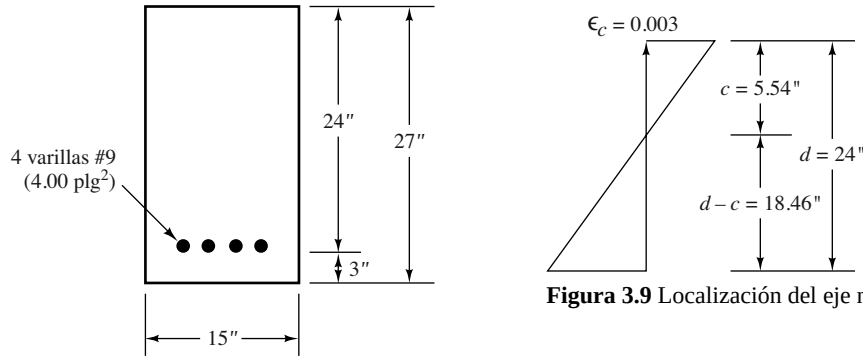
Figura 3.8 Sección transversal de la viga del Ejemplo 3.2
