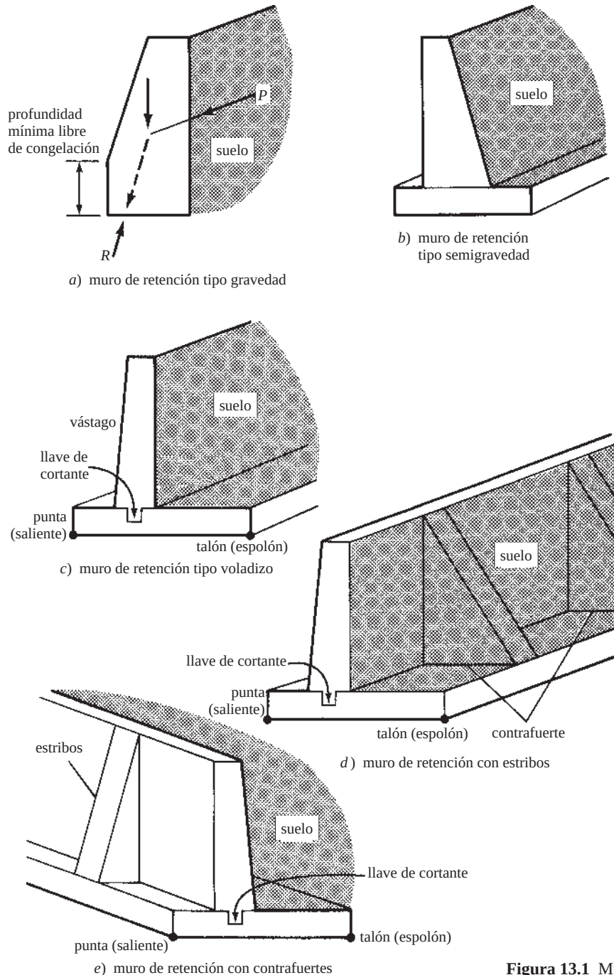
Figura 13.1 Muros de retención.
