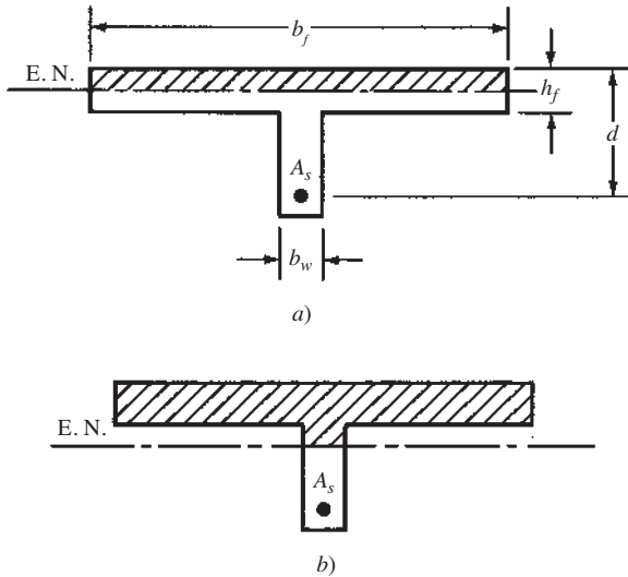
Figura 5.2 Ubicaciones de los ejes neutrales.
