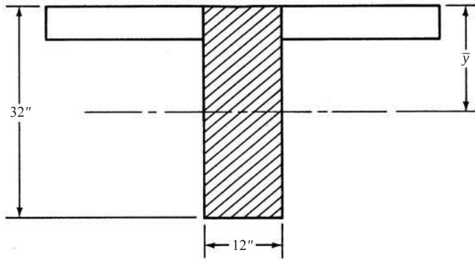
Figura 6.10 Centroides de la sección sin agrietar para el momento negativo en el Ejemplo 6.2.
