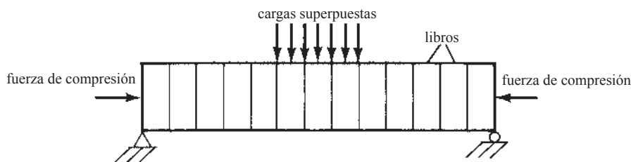
Figura 19.1 Presfuerzo.
