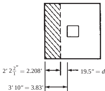
Figura 12.11 Cortante en una dirección para el Ejemplo 12.2.
