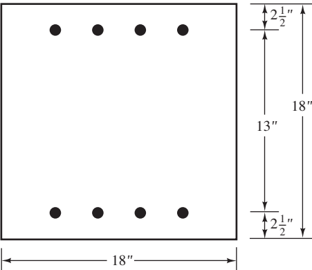
Figura 11.8 Sección transversal de la columna del Ejemplo 11.4.
