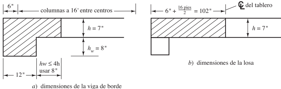
Figura 16.7 Secciones transversales de la viga de borde y de la losa.
