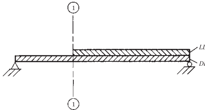
Figura 14.22 Posición de la carga viva para el cortante máximo en la sección 1-1.
