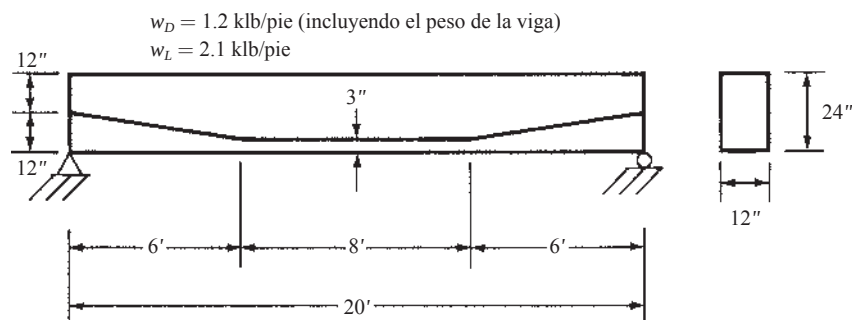
Figura 19.13 Información del Ejemplo 19.5.
