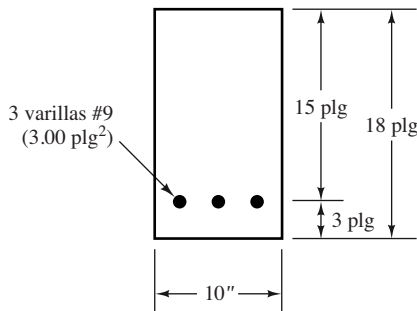
Figura 3.11 Sección transversal de la viga el Ejemplo 3.4.
