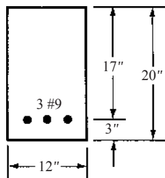
Figura 6.5 Sección transversal de la viga del Ejemplo 6.1.
