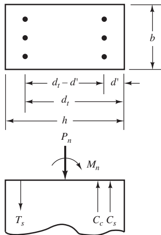
Figura 10.26 Notación usada para la sección transversal de una columna.
