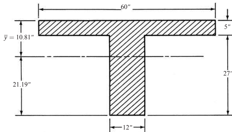
Figura 6.8 Centroides de la sección no agrietada en el Ejemplo 6.2.
