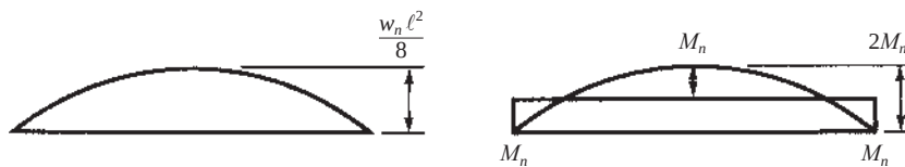
Figura 14.13 Determinación del M_n requerido en una viga doblemente empotrada con un mecanismo de formación de articulaciones.
