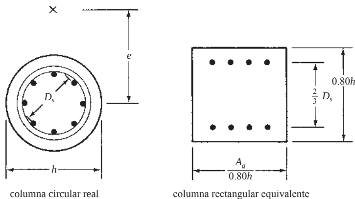
Figura 10.9 Reemplazo de una columna circular por una rectangular equivalente.
