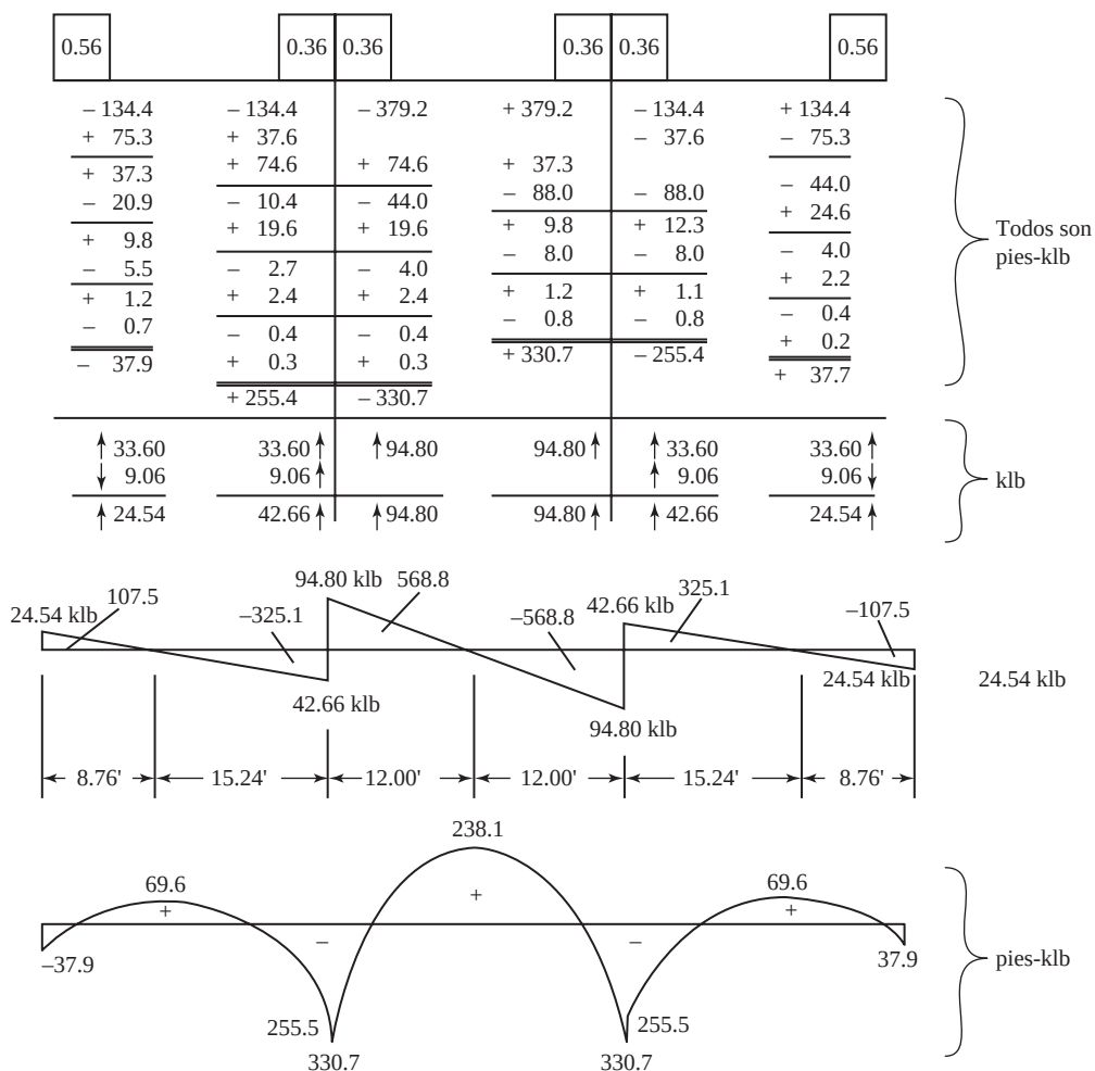
Figura 14.28 Resultados de la distribución de momentos del Ejemplo 14.2
