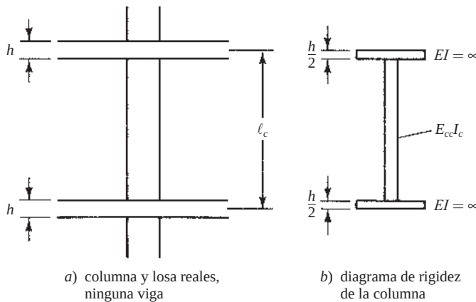
Figura 17.7 Columna equivalente.
