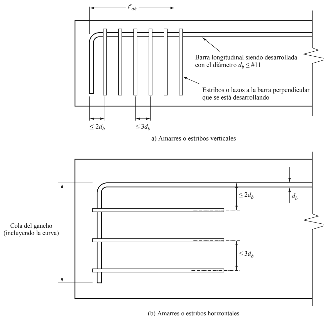
Figura 7.14 Los amarres o estribos paralelos a la varilla que se está desarrollando a lo largo de la longitud de la prolongación terminal de un gancho de 90^\circ más el doblez cumplen con el multiplicador \psi_r = 0.8 . Los estribos o amarres mostrados pueden ser verticales u horizontales. [Código 318 del ACI, Figura R25.4.3.2a) y b)]. Fuente: Reproducido con autorización del American Concrete Institute .
