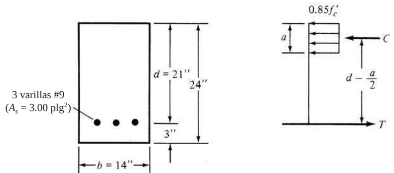
Figura 2.12 Sección transversal de la viga del Ejemplo 2.8.
