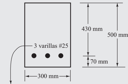
Figura 2.15 Sección transversal de la viga del Ejemplo 2.10.
