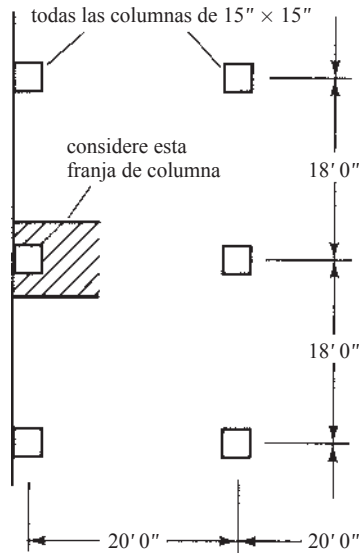
Figura 16.22 Dimensiones de la losa plana del Ejemplo 16.5.
