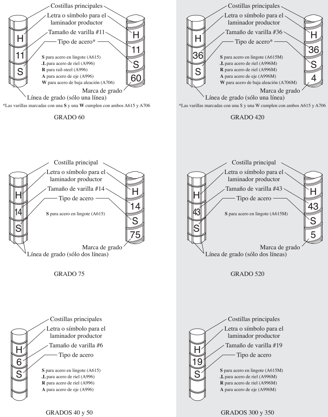
Figura 1.4 Marcas de identificación para varillas estándar ASTM. (Cortesía del Concrete Reinforcing Steel Institute.)
