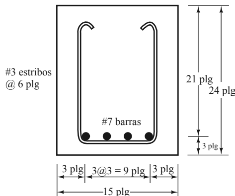
Figura 7.9 Sección transversal de la viga del Ejemplo 7.3.
