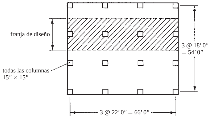
Figura 17.9 Placa plana del Ejemplo 17.2.
