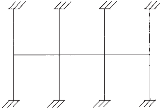
Figura 16.2 Método del marco equivalente.
