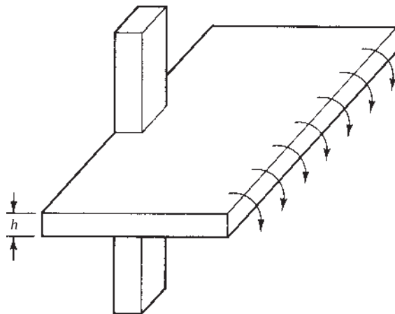
Figura 16.20 Ilustración que muestra la necesidad de la transferencia de los momentos a las columnas.
