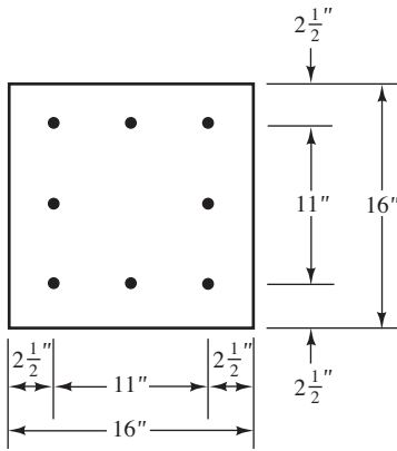
Figura 10.18 Sección transversal de la columna del Ejemplo 10.4.
