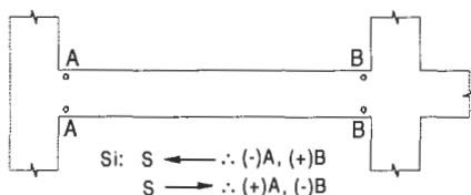
SECCIONES CRITICAS PARA CARGAS SISMICAS
