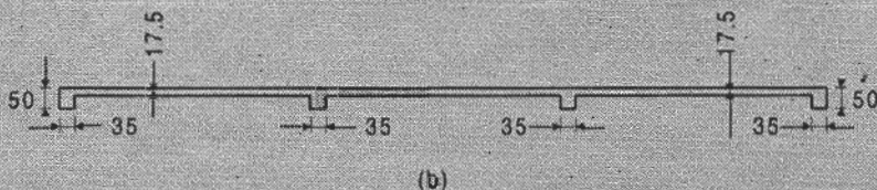
Figura, losa de piso armada en dos direcciones con vigas en los ejes de columnas: (a) Planta parcial del piso; (b) Sección X-X (la sección Y-Y es similar).
