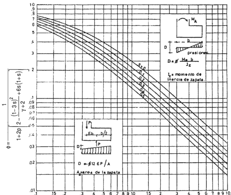
Fig. 1: Gráfico para la determinación de presiones bajo la cimentación
