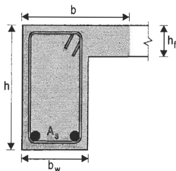
Sección transversal de viga T
