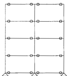
a) Viga Debil - Columna Fuerte
