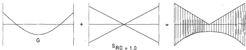
Envolvente usando fuerzas sísmicas sin reducir
